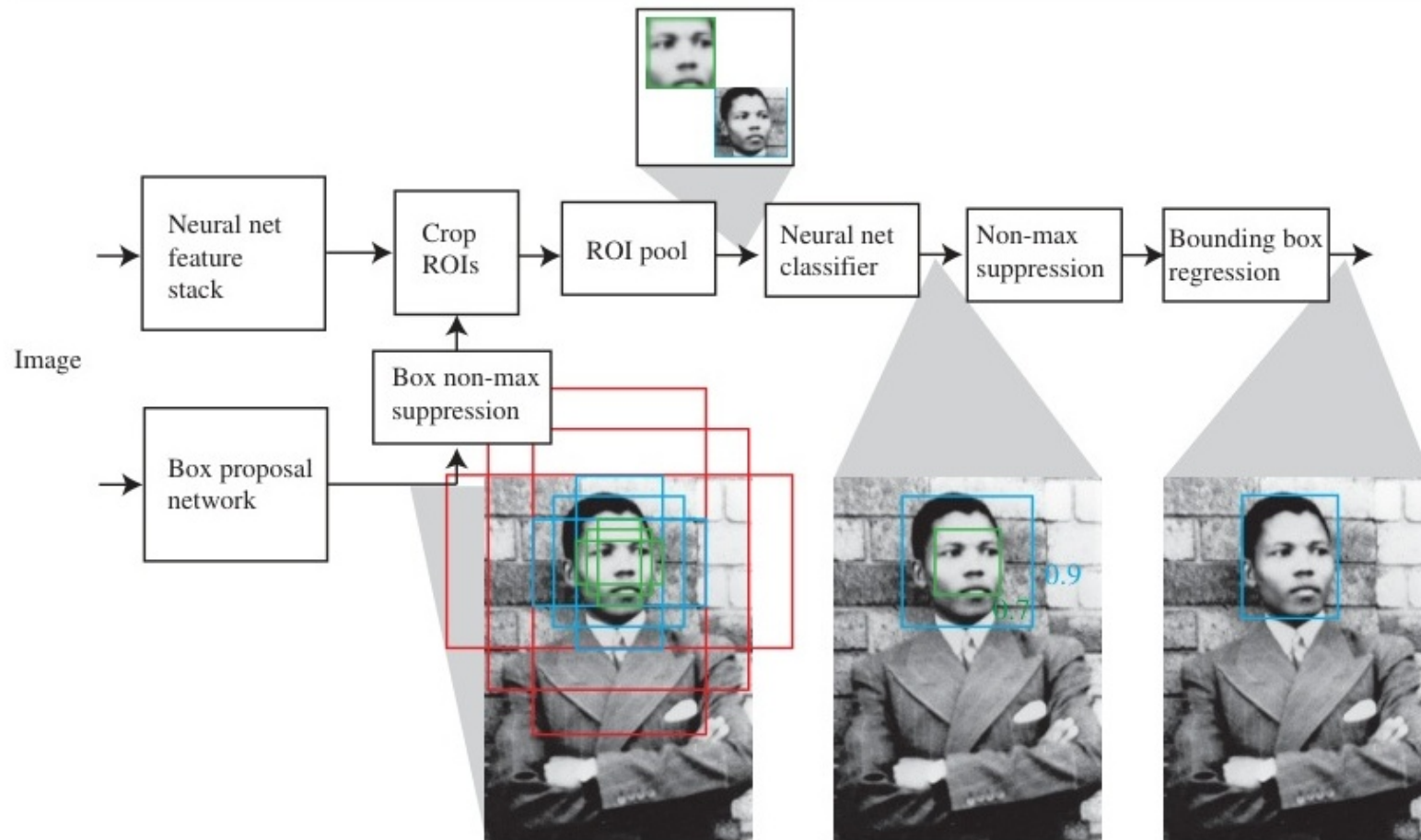
Figure 13: Sơ đồ kiến trúc Faster R-CNN quét các hộp neo để khoanh vùng và phân loại khuôn mặt.
