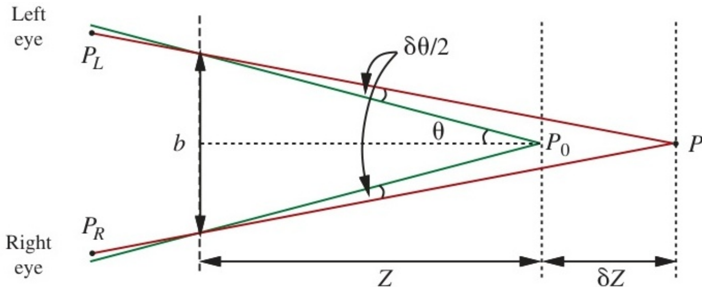
Figure 15: Mối quan hệ hình học giữa điểm hội tụ, độ lệch góc chiếu và chiều sâu Z trong thị giác âm nổi.
