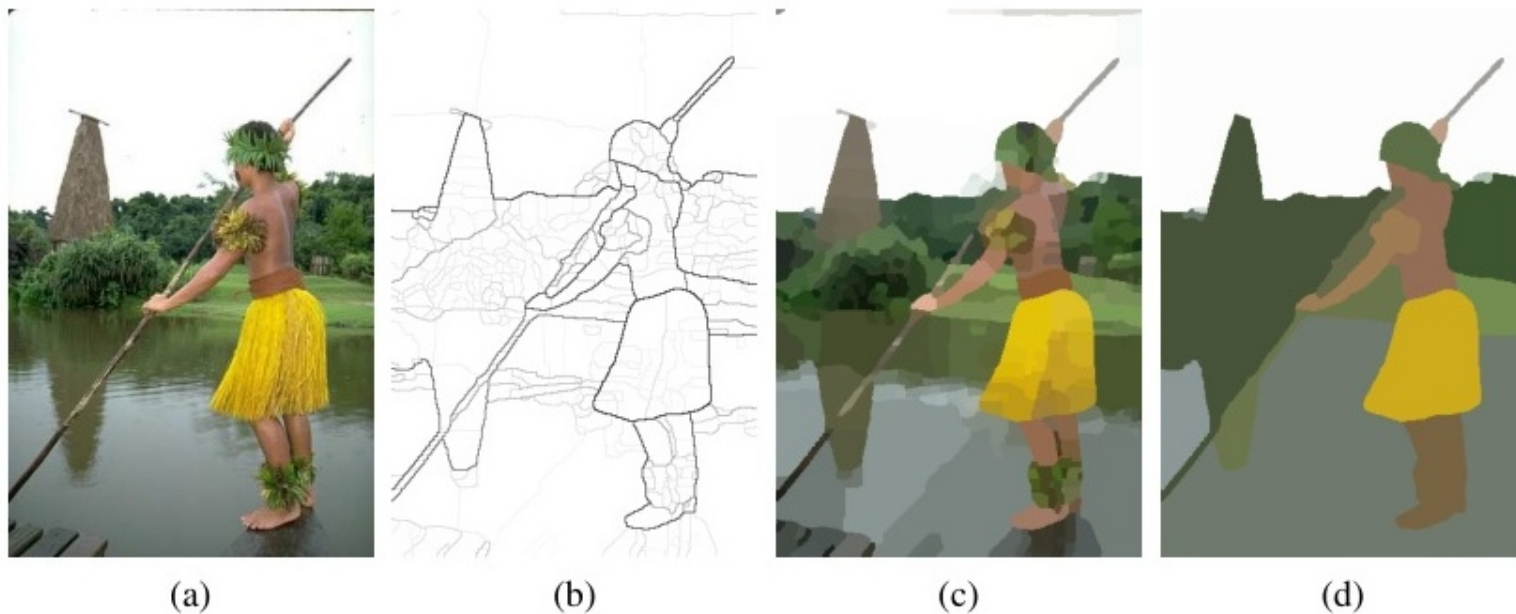
Figure 10: Biểu diễn các đường biên P_b và kết quả phân đoạn ảnh tinh (nhiều vùng) và thô (ít vùng).
