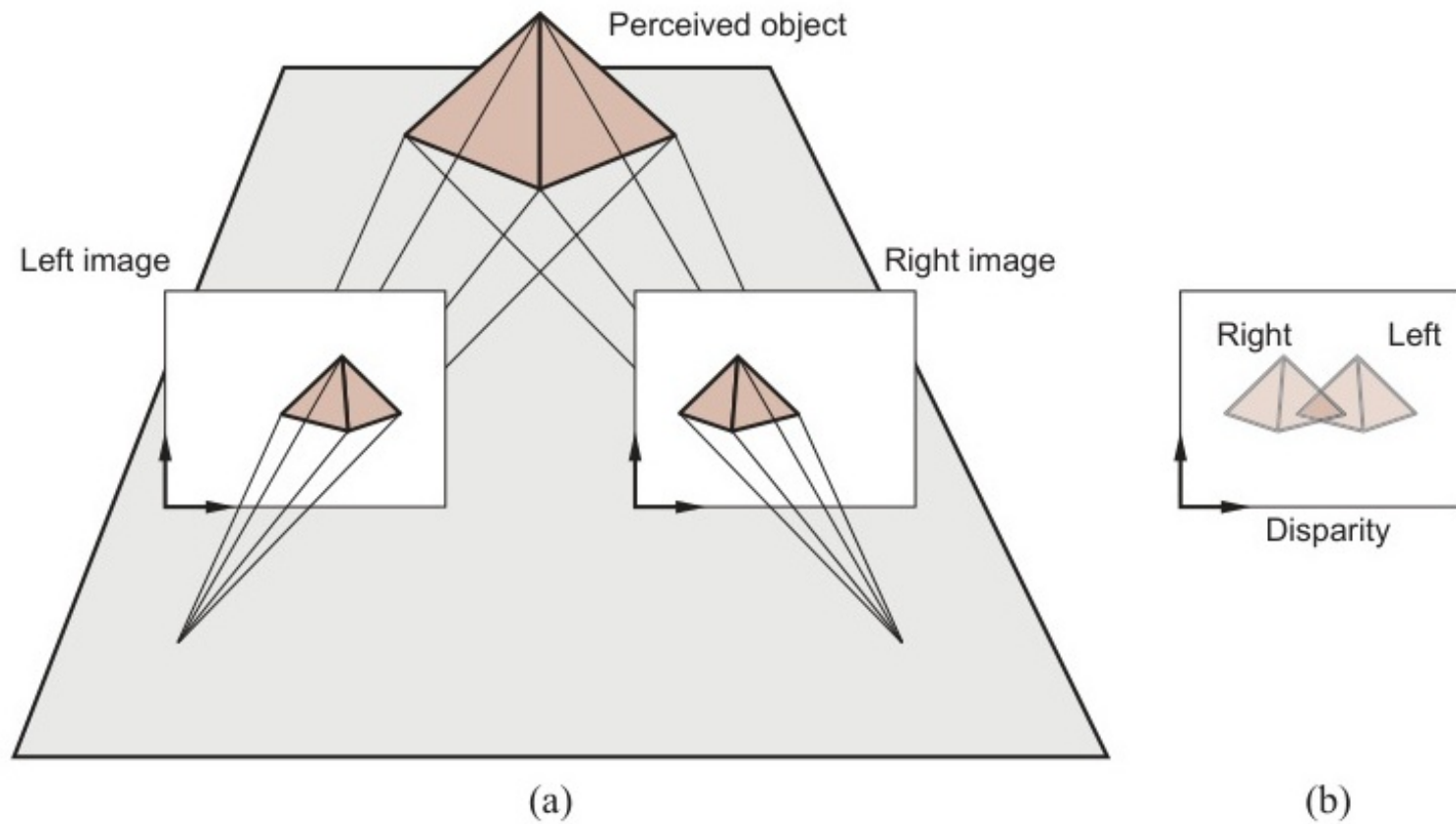
Figure 14: Sự dịch chuyển tương đối của đặc trưng trên mặt phẳng ảnh tùy thuộc vào khoảng cách tới camera.
