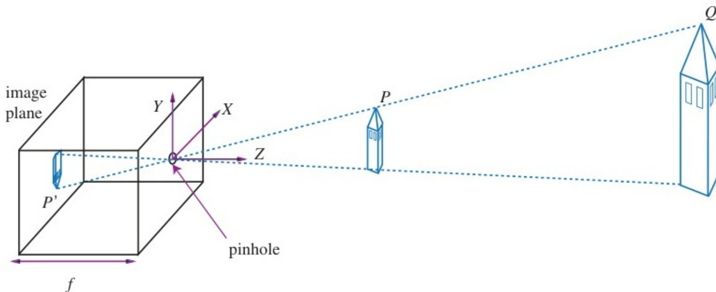
Figure 2: Nguyên lý máy ảnh lỗ kim: Ánh sáng từ nguồn bị thu hẹp lại tạo ảnh lộn ngược trên mặt phẳng.
