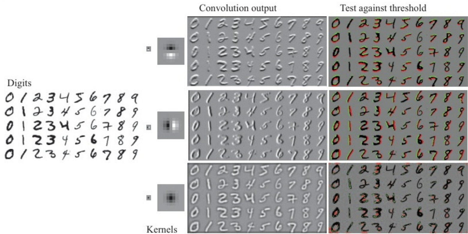
Figure 12: Các bộ lọc kernel phân tách đường nét thành phần của một bức ảnh chữ số viết tay.
