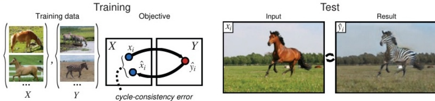
Figure 25: CycleGAN phù phép hóa tiết ngựa vằn lên một con ngựa thường nhờ học tính phân bố miền.
