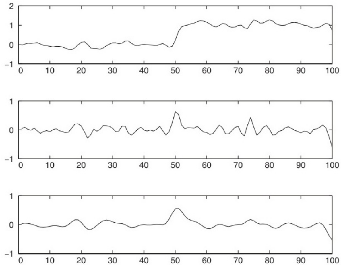
Figure 7: Tác dụng của việc làm mịn bằng Gauss trước khi lấy đạo hàm để loại bỏ các điểm nhiễu cục bộ.
