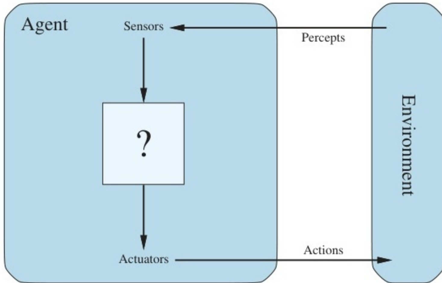
Figure 2.1: Mô hình Tác nhân tương tác với môi trường thông qua Cảm biến và Cơ cấu chấp hành.
