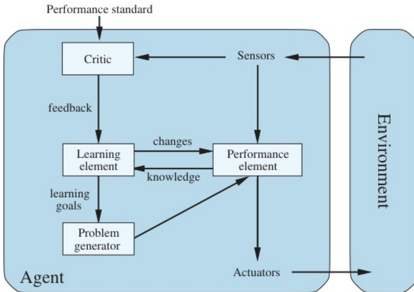
Figure 2.15: Mô hình cấu trúc chung cho Tác nhân có khả năng học thuật.
