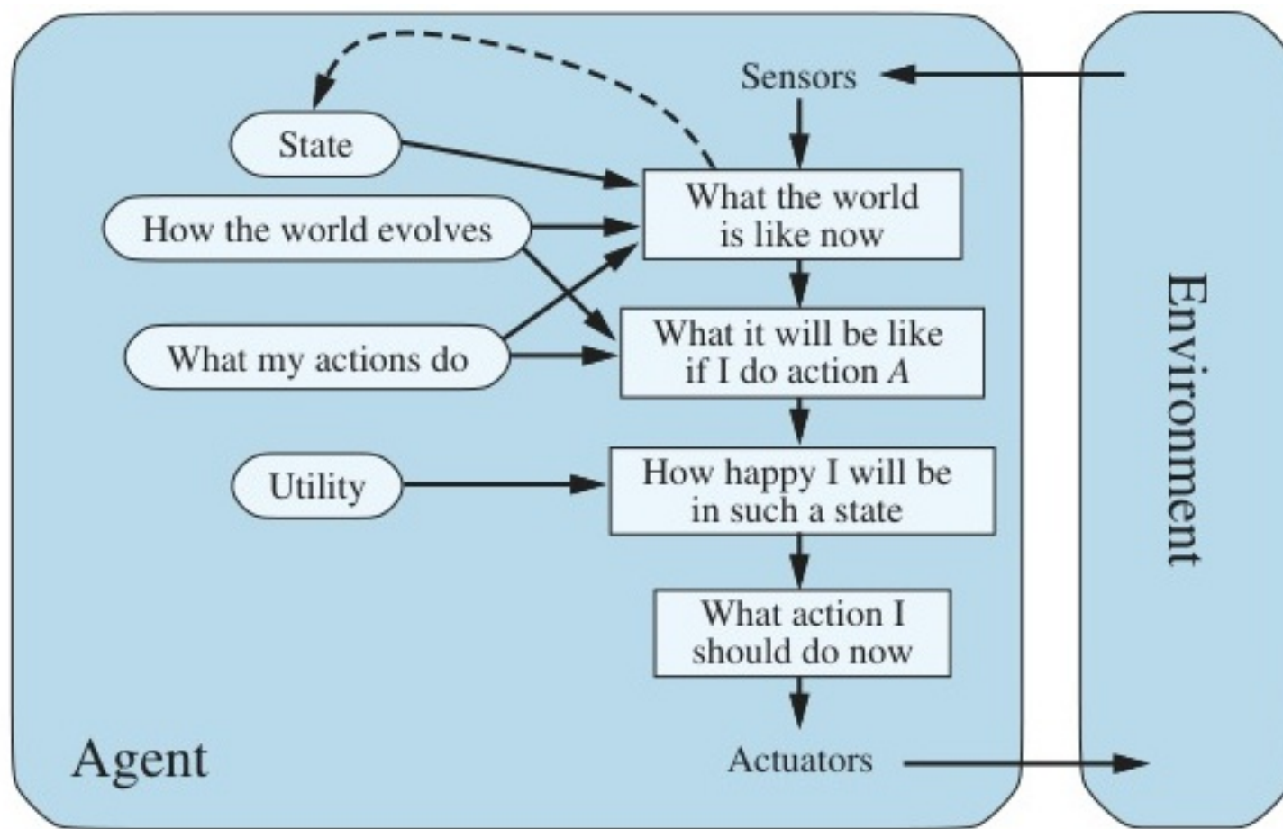
Figure 2.14: Mô hình Tác nhân dựa trên tiện ích (Utility-based agent).
