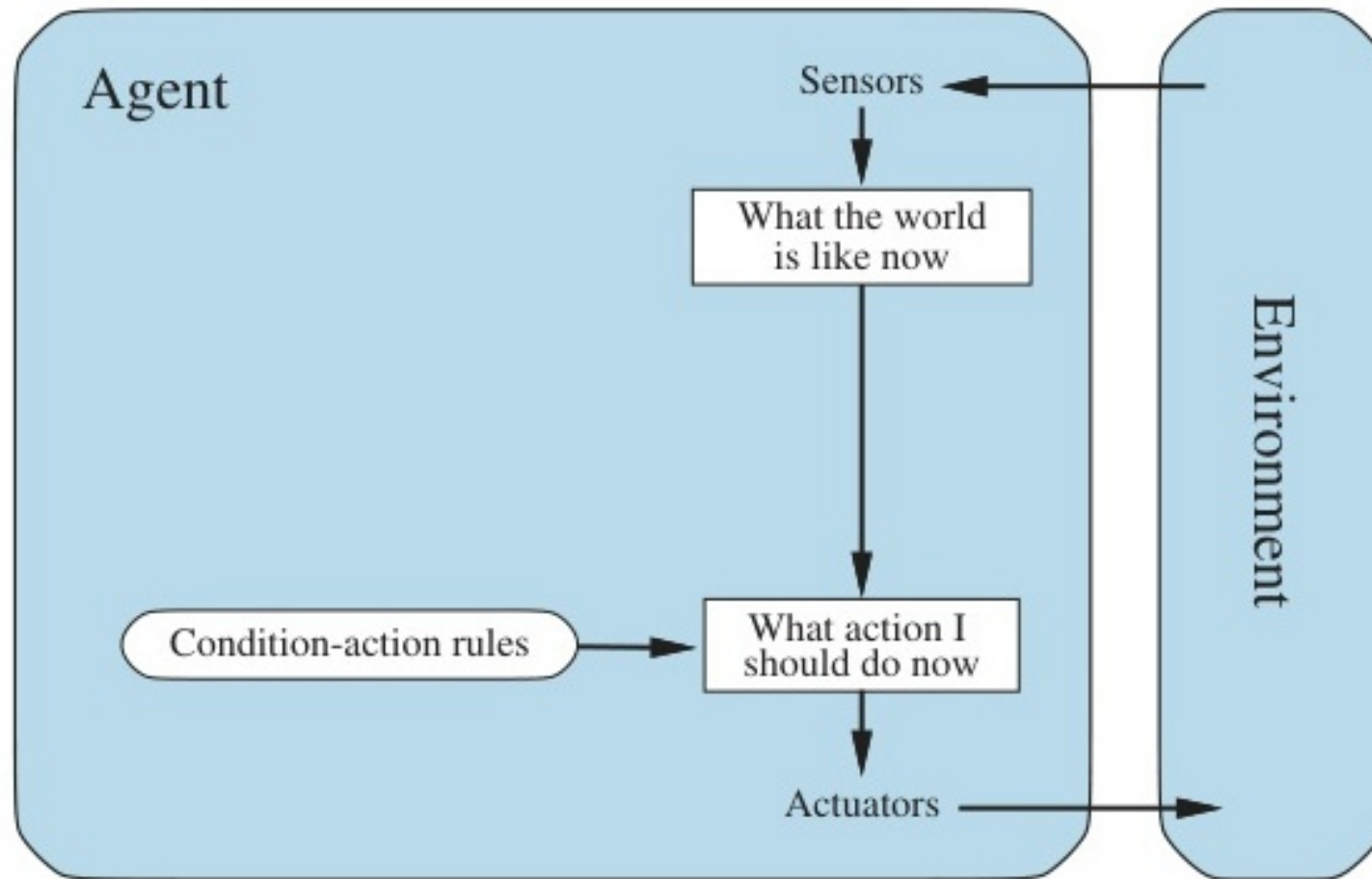
Figure 2.9: Mô hình Tác nhân phản xạ đơn giản (Simple reflex agent).
