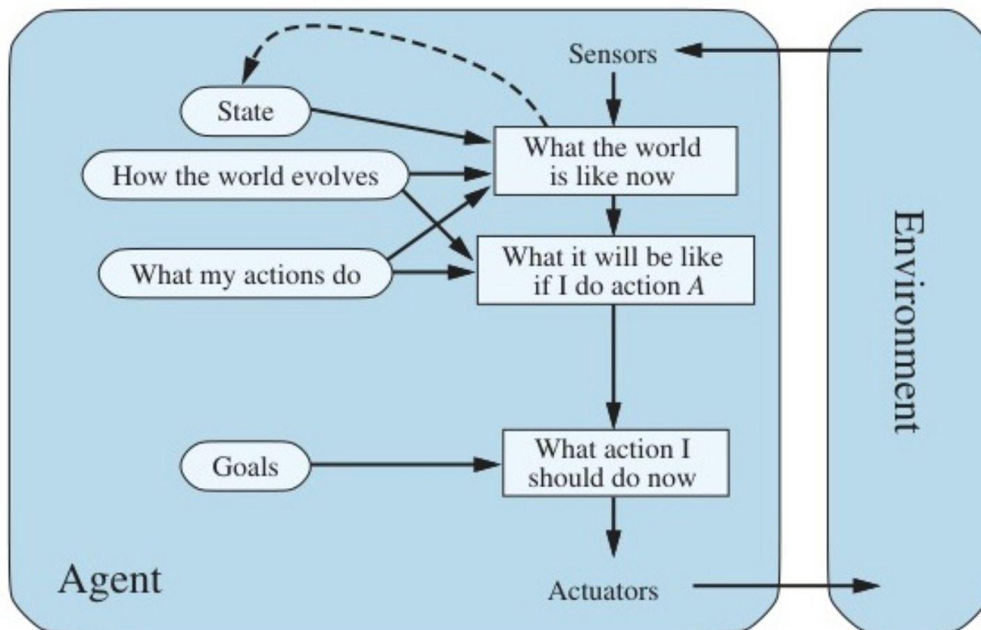
Figure 2.13: Mô hình Tác nhân dựa trên mục tiêu (Goal-based agent).
