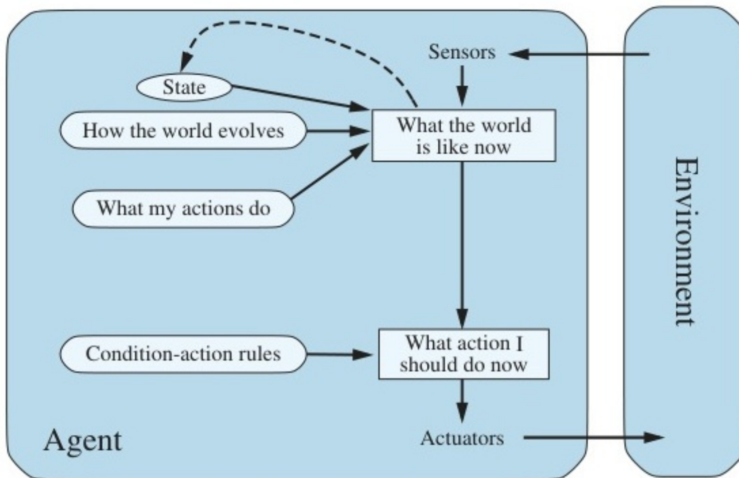
Figure 2.11: Mô hình Tác nhân phản xạ dựa trên mô hình (Model-based reflex agent).
