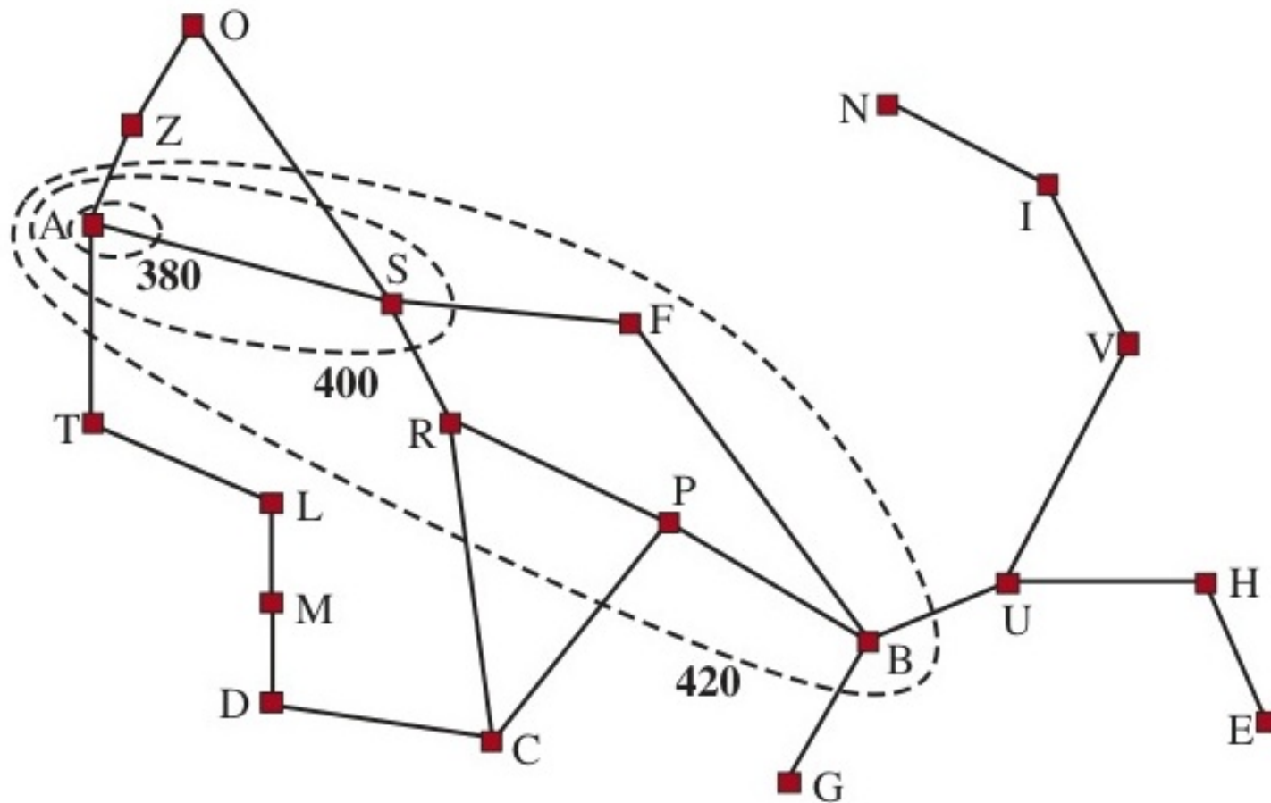
Figure 3.20: Các đường đồng mức f(n) trên bản đồ Romania.
