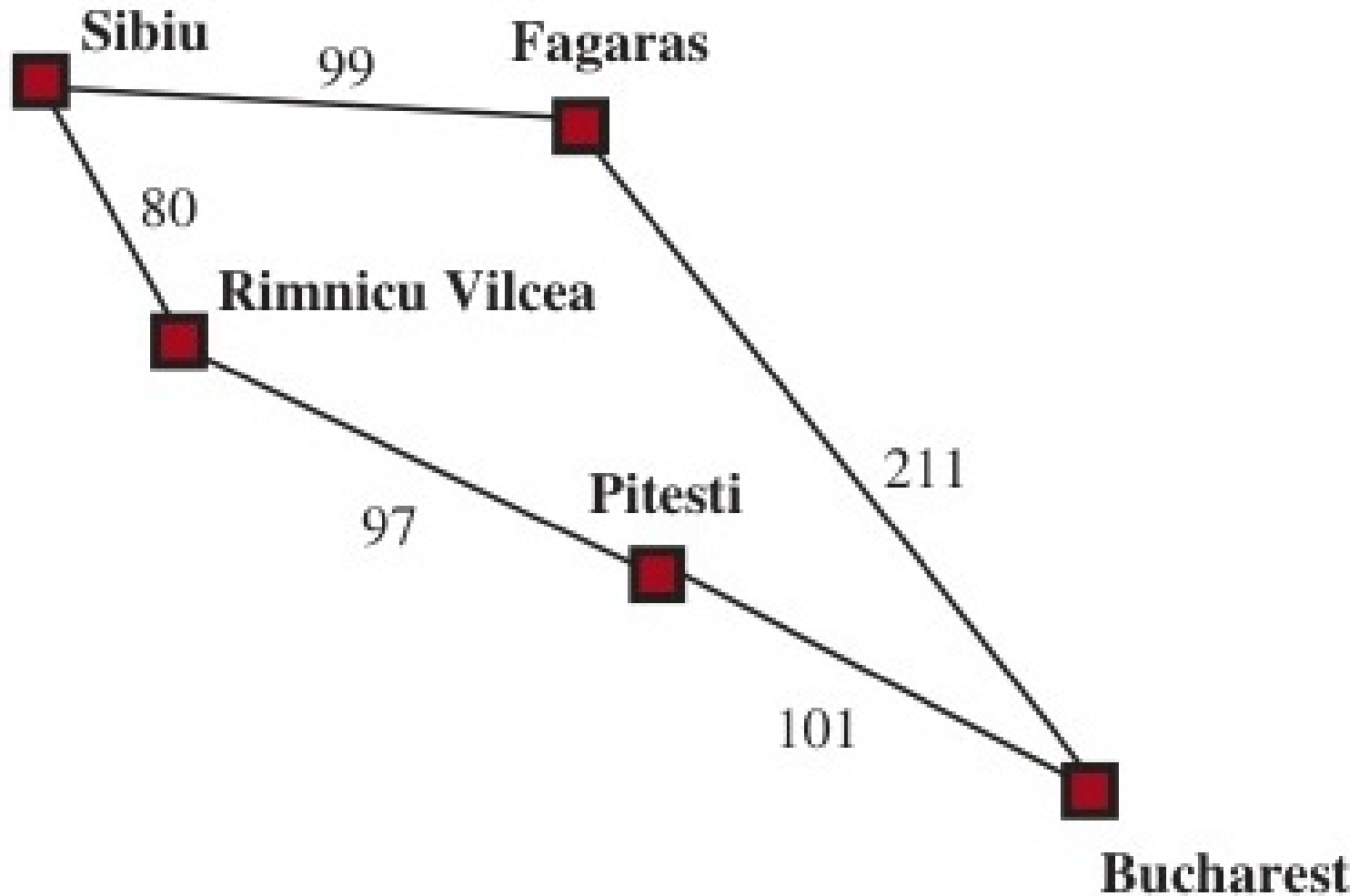
Figure 3.10: Một phần không gian trạng thái ở Romania để minh họa thuật toán UCS.
