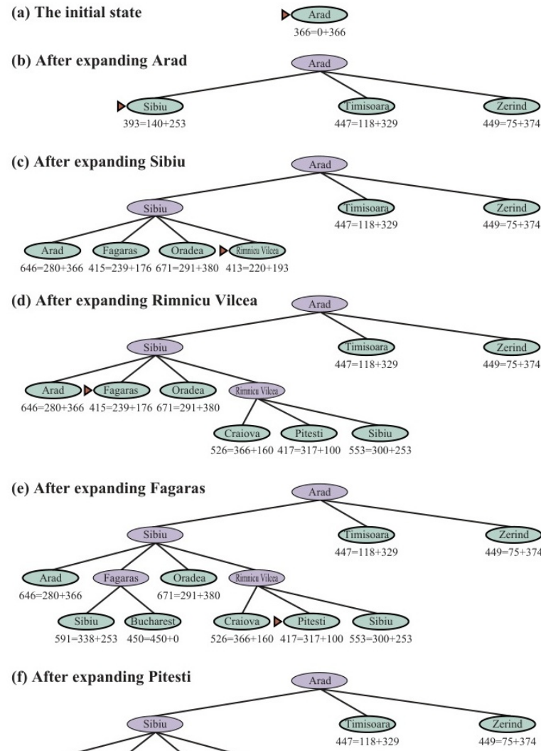
Figure 3.18: Quá trình mở rộng bằng A* Search, cân bằng giữa g(n) và h(n) .
