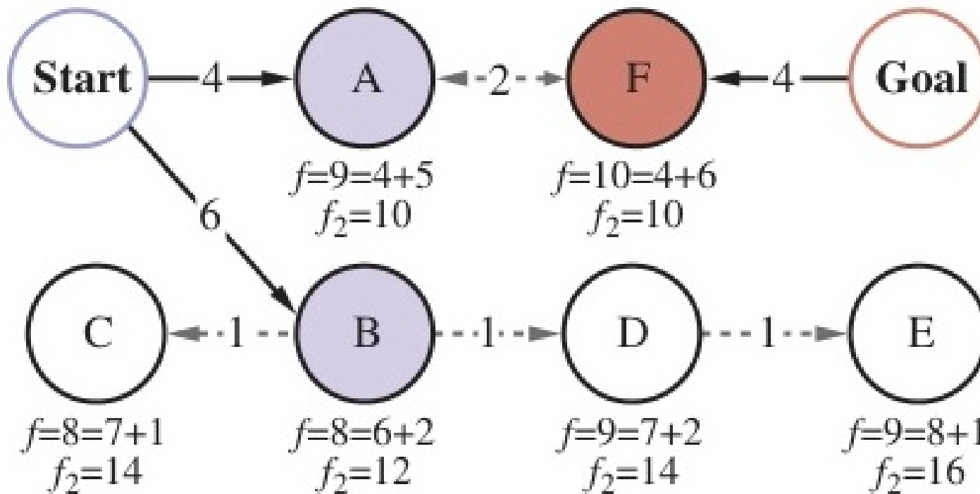
Figure 3.24: Đồ thị tìm kiếm hai chiều: Mở rộng đồng thời từ điểm xuất phát và mục tiêu.
