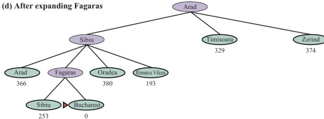
Figure 3.17: Quá trình tìm đường bằng thuật toán Greedy Best-First Search.
