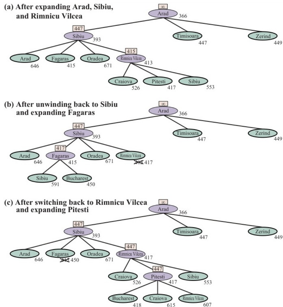
Figure 3.23: Các giai đoạn mở rộng nút của thuật toán RBFS trên bản đồ Romania.
