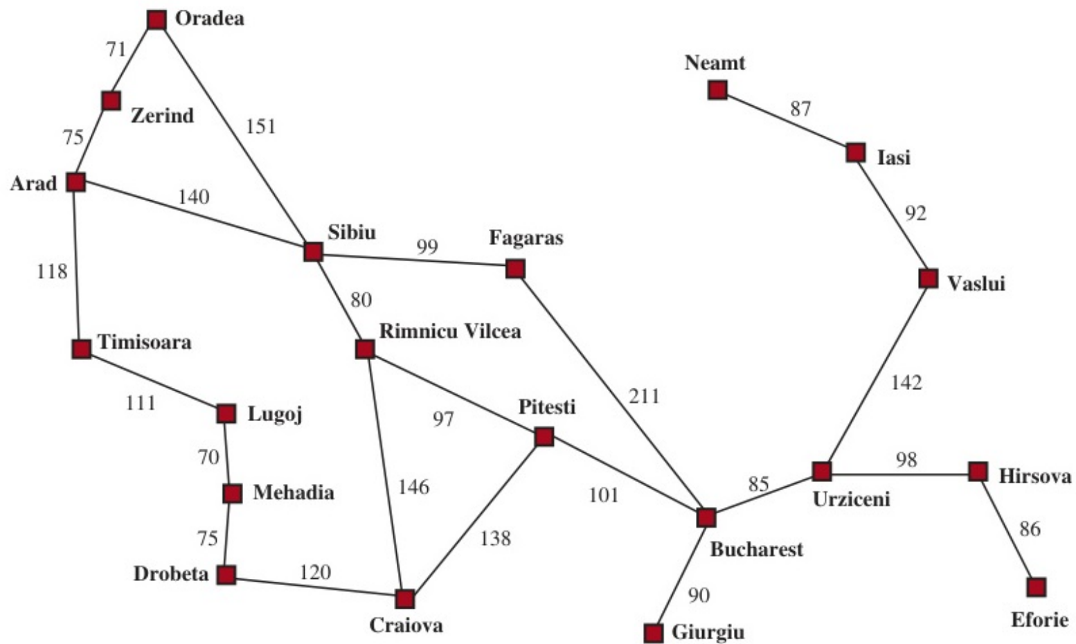
Figure 3.1: Bản đồ Romania với khoảng cách giữa các thành phố.
