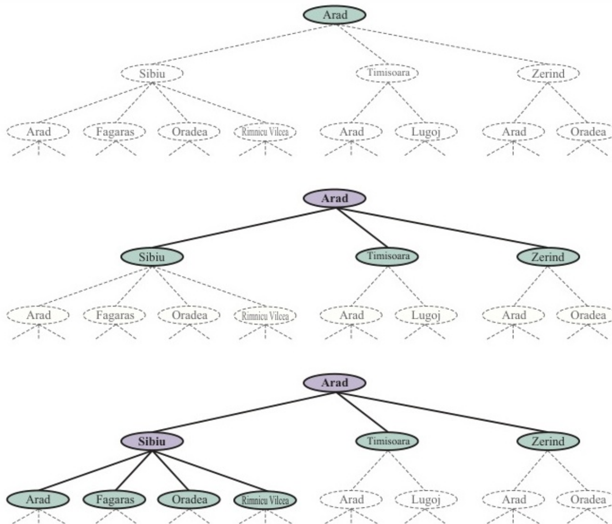
Figure 3.4: Quá trình mở rộng cây tìm kiếm từ Arad đi Bucharest.
