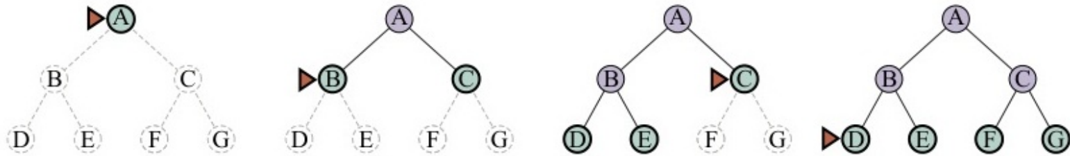
Figure 3.8: Quá trình mở rộng nút trong BFS trên cây nhị phân.
