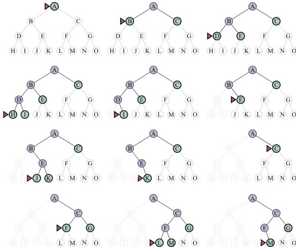
Figure 3.12: Quá trình tìm kiếm theo chiều sâu đầu tiên trên cây nhị phân.
