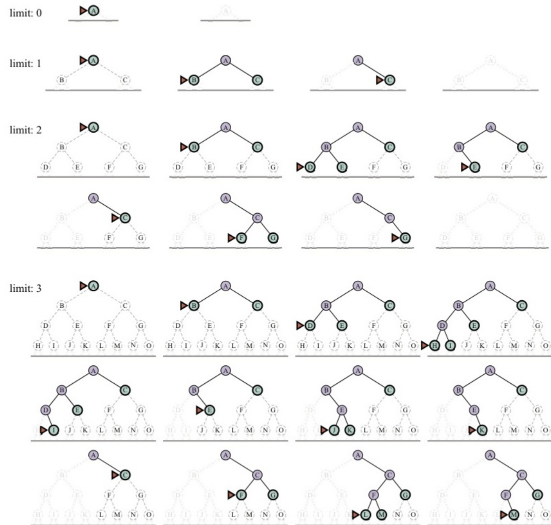
Figure 3.16: Bốn lần lặp của thuật toán IDS trên cây nhị phân.
