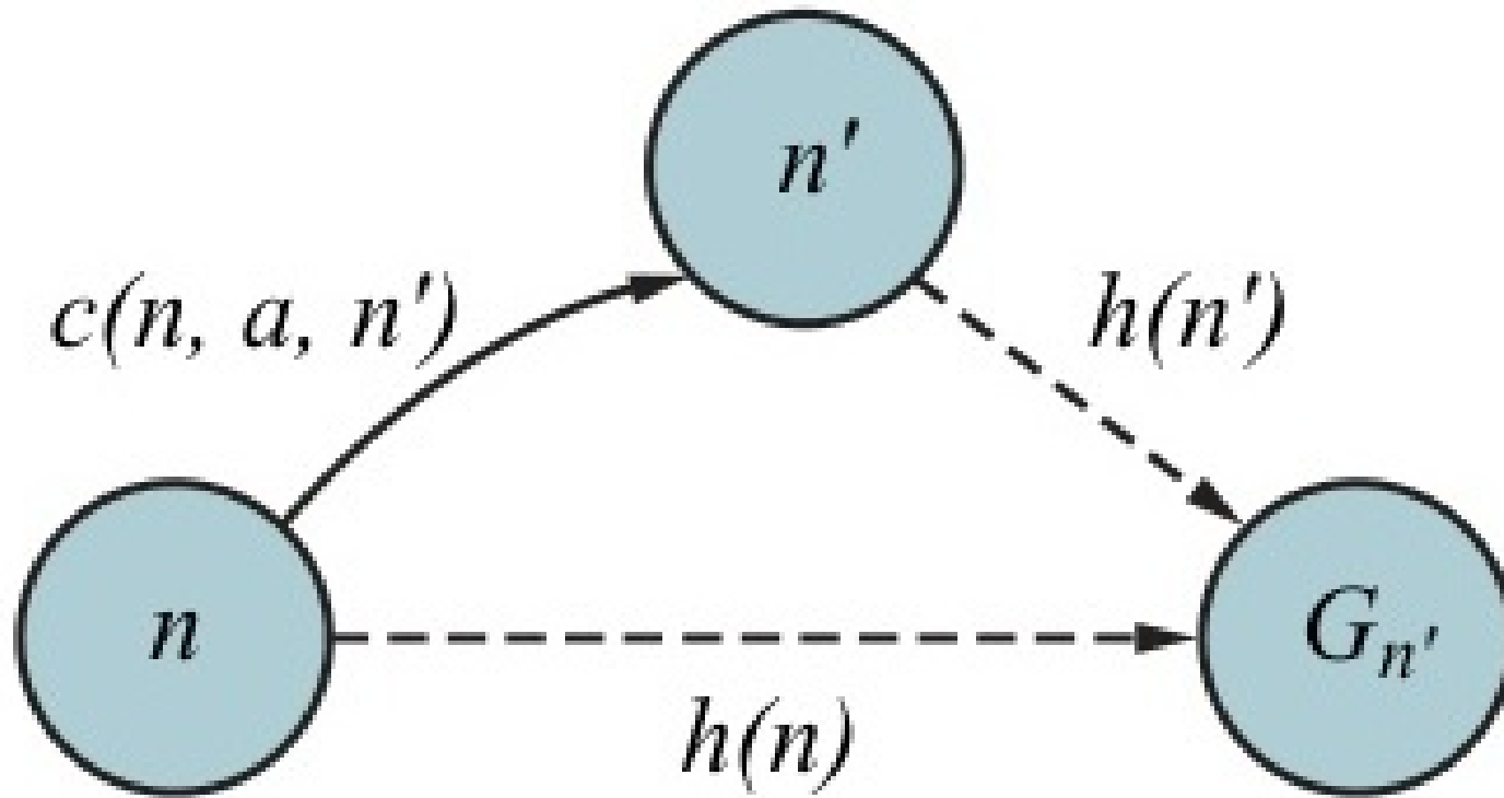
Figure 3.19: Bất đẳng thức tam giác minh họa tính nhất quán (Consistency).
