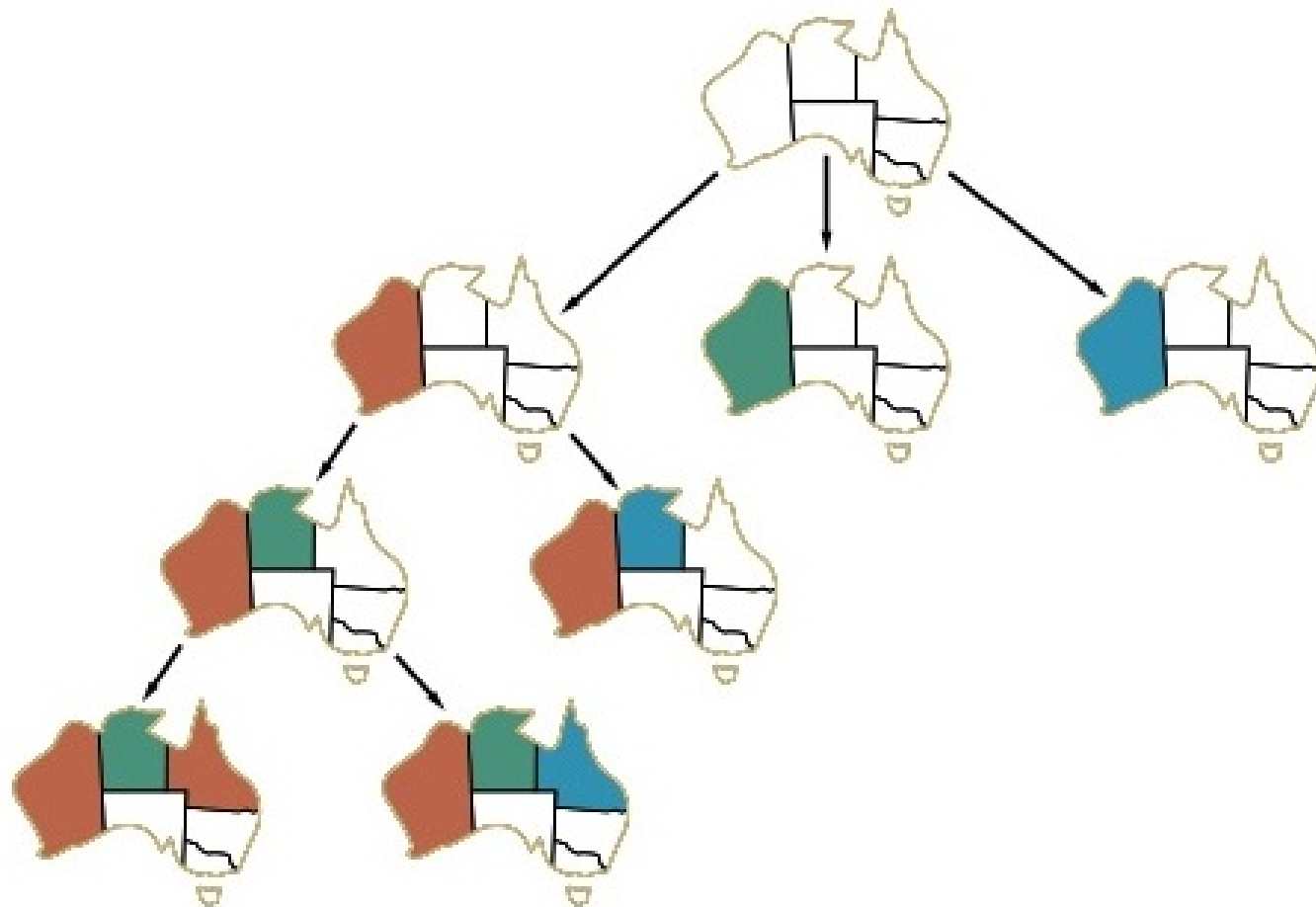
Figure 5.6: Mô phỏng Tìm kiếm Quay lui qua cây quyết định gán giá trị màu sắc.
