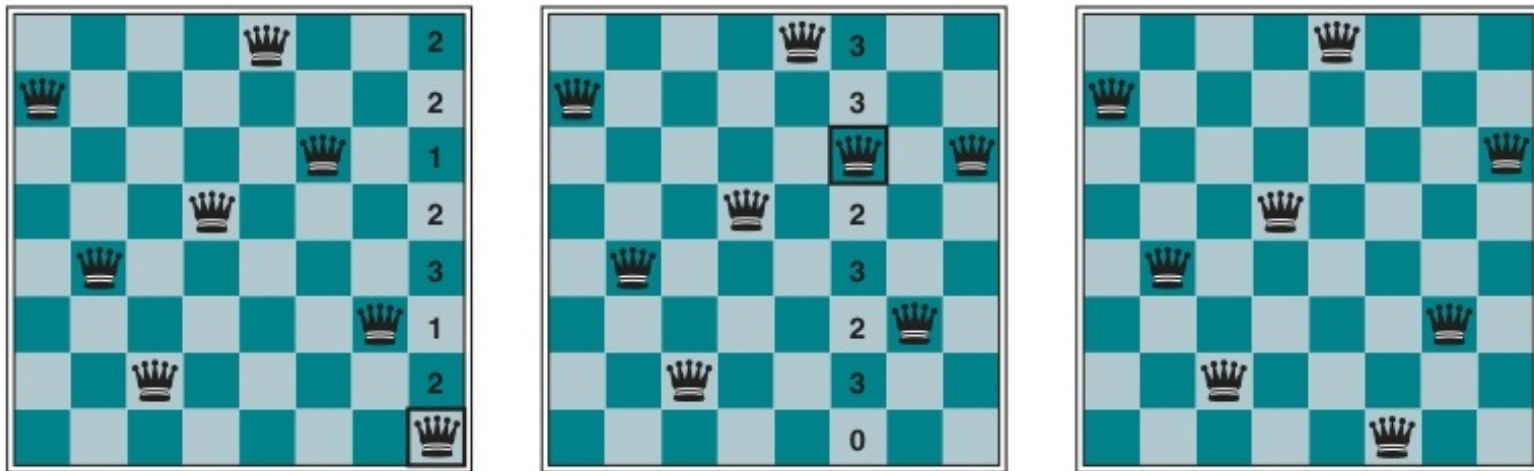
Figure 5.9: Giải pháp hai bước sử dụng mâu thuẫn tối thiểu cho bài toán 8 con hậu.
