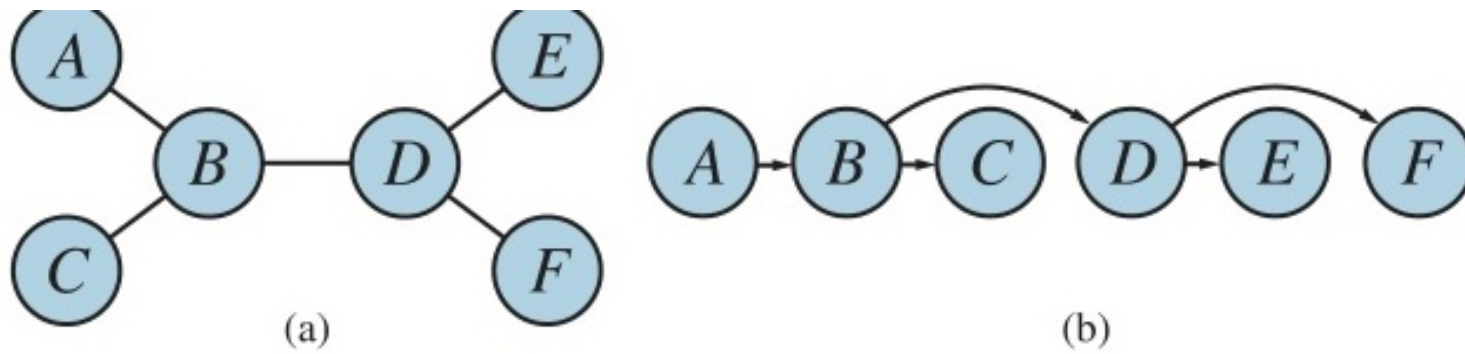
Figure 5.10: Đồ thị ràng buộc của một CSP có cấu trúc cây.
