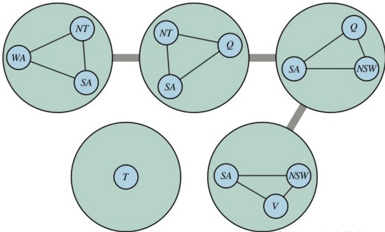
Figure 5.13: Một phân rã cây (Tree decomposition) của đồ thị ràng buộc bản đồ Úc.
