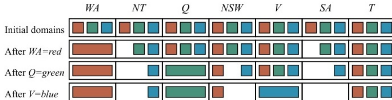
Figure 5.7: Minh họa quá trình Forward Checking loại bỏ trước các giá trị tương lai.
