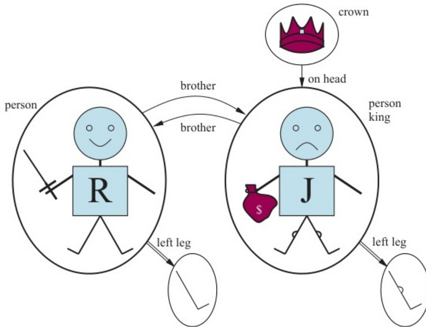
Figure 8.3: Một mô hình chứa 5 đối tượng (King John, Richard...), 2 quan hệ hai ngôi, 3 quan hệ một ngôi, và một hàm.
