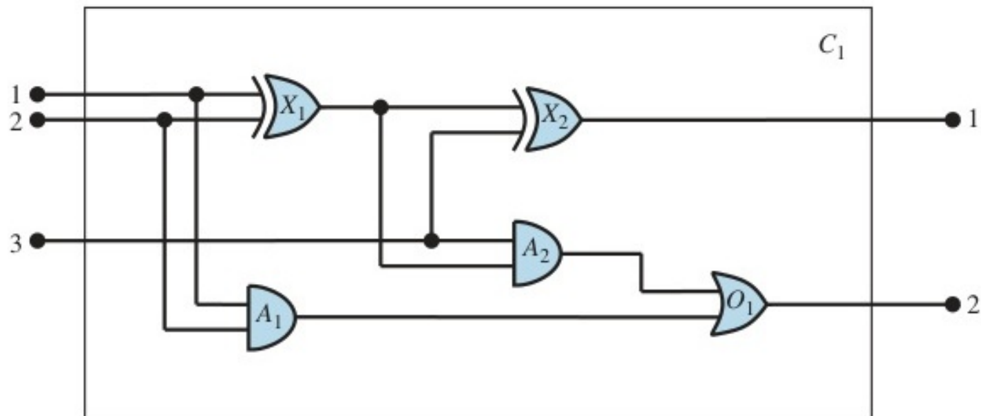
Figure 8.6: Một mạch kỹ thuật số (bộ cộng đầy đủ 1-bit), có thể được biểu diễn và chẩn đoán lỗi bằng FOL.
