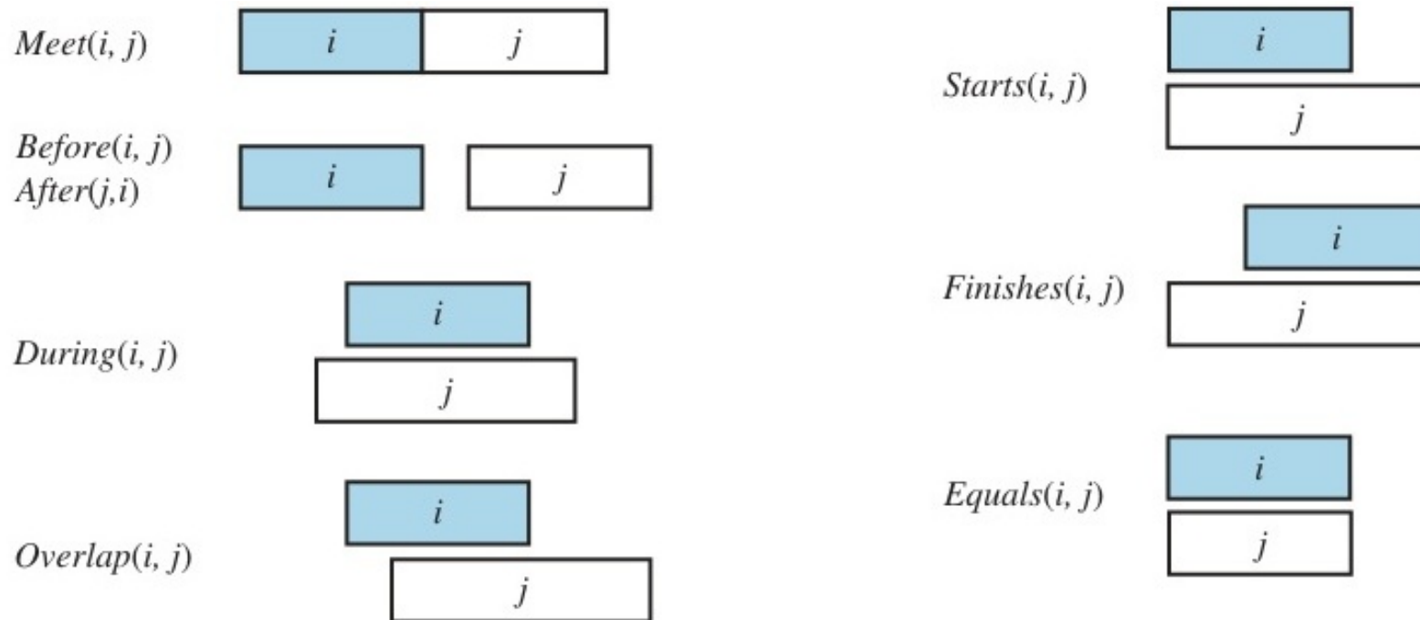
Figure 10.2: Các vị từ trên khoảng thời gian (Meet, Before, After, During...) giúp định vị sự kiện.
