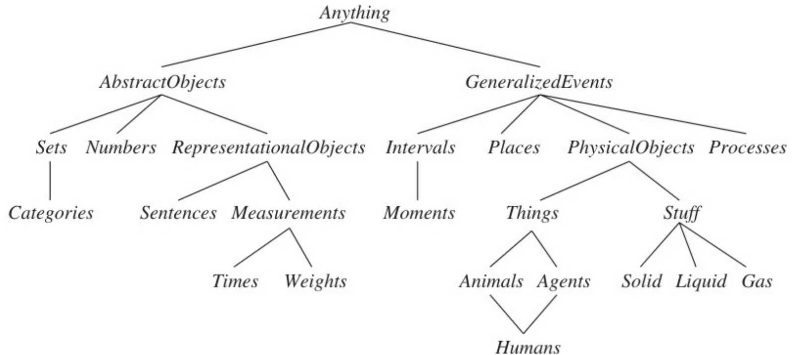
Figure 10.1: Sơ đồ phân loại tổng quát (Upper Ontology): Chia mọi thứ thành Đối tượng trừu tượng, Đối tượng vật lý, Không gian, Thời gian và Sự kiện.
