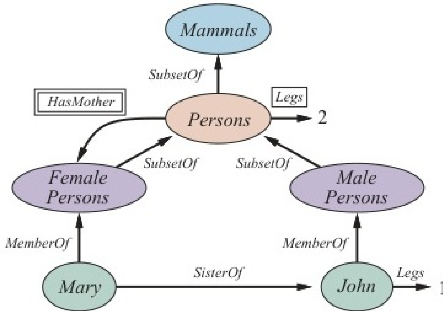
Figure 10.4: Mạng ngữ nghĩa với bốn đối tượng (John, Mary, 1 và 2) và các phạm trù, liên kết với nhau bằng các cung.
