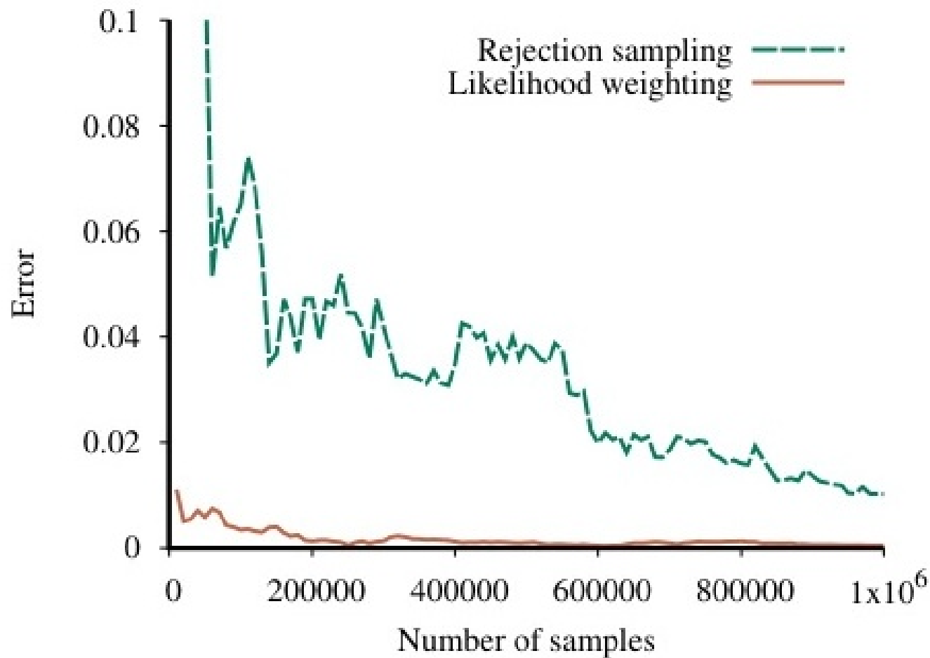
Figure 13.11: Đồ thị biểu diễn sai số theo số lượng mẫu của hai phương pháp Rejection Sampling và Likelihood Weighting.
