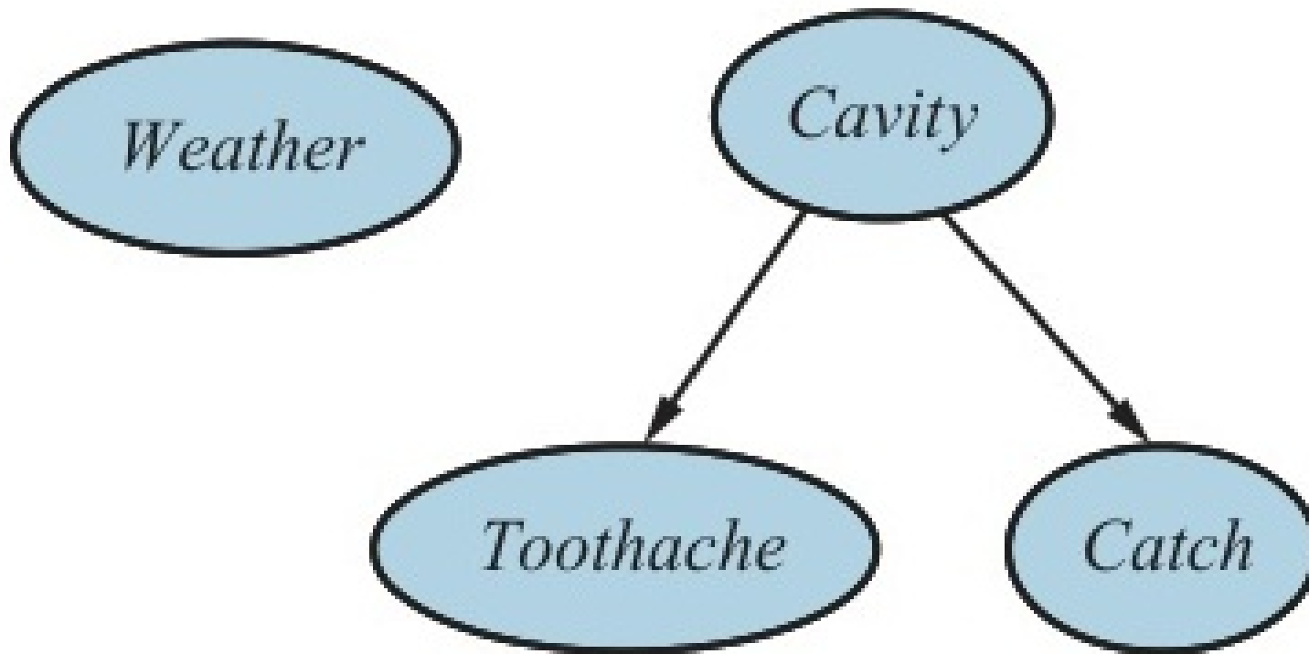
Figure 13.1: Mô hình phụ thuộc nhân quả giữa Thời tiết ( Weather ), Sâu răng ( Cavity ), Đau răng ( Toothache ) và Catch.
