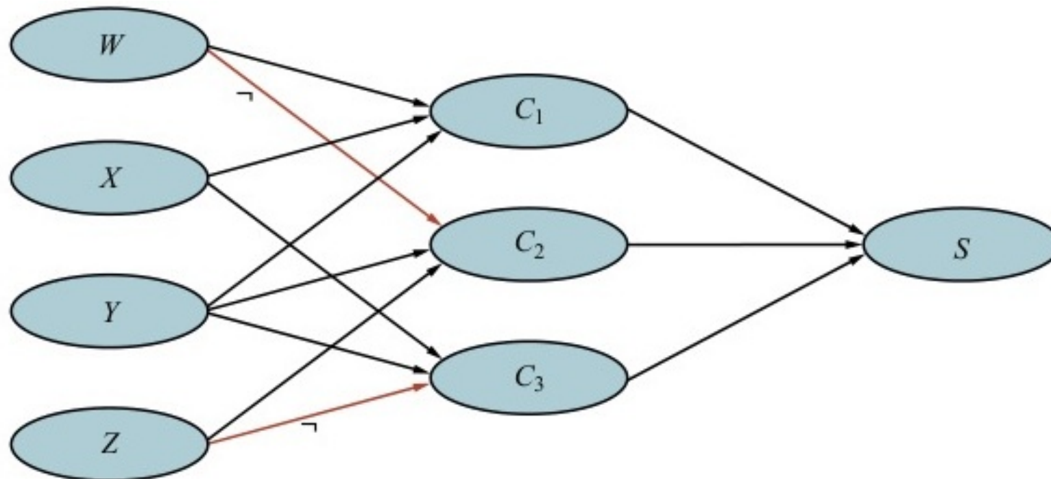
Figure 13.6: Mã hóa bài toán 3-SAT dưới dạng mạng Bayes, minh chứng tính chất NP-hard của bài toán suy luận xác suất.
