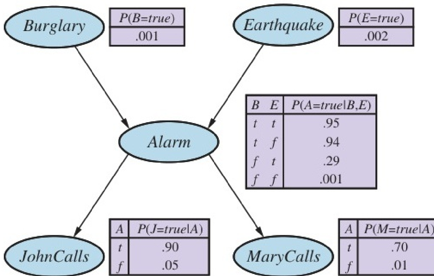
Figure 13.2: Một mạng Bayes diễn hình, hiển thị cả cấu trúc topo và các bảng xác suất có điều kiện (CPT) của bài toán báo trộm.
