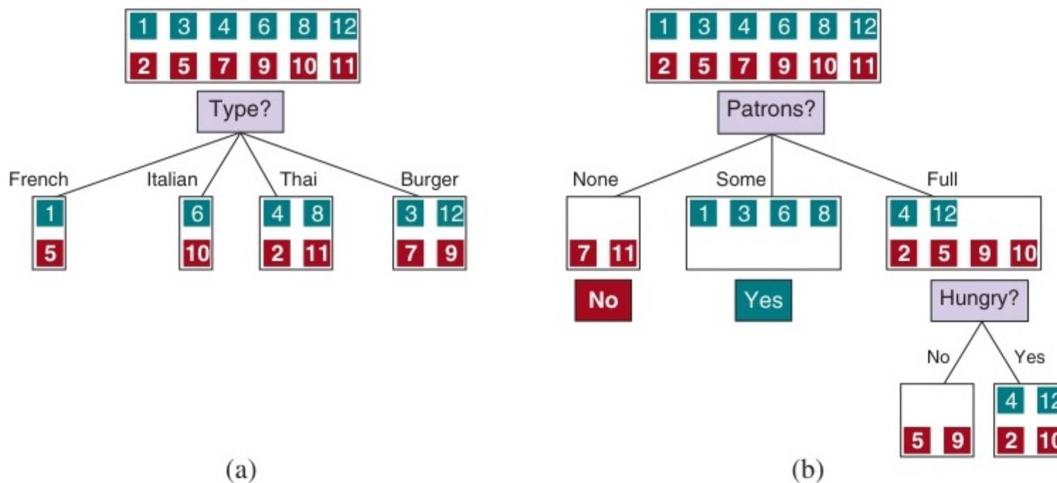
Figure 19.3: Đánh giá khả năng phân tách của các thuộc tính để tìm ra thuộc tính tốt nhất đưa lên Nút Gốc.
