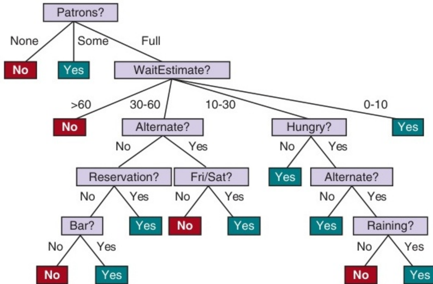
Figure 19.2: Một cây quyết định mẫu để quyết định xem có nên đợi bàn hay không.
