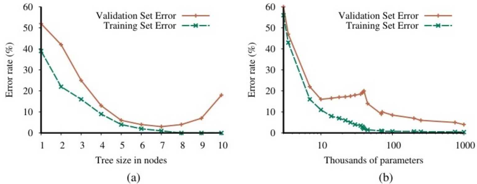
Figure 19.4: Hiện tượng Khớp quá mức (Overfitting): Tỷ lệ lỗi trên tập Validation (đường đỏ) bắt đầu tăng vọt khi cây quá sâu.
