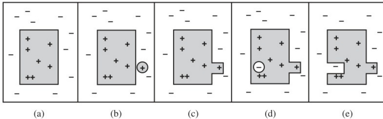
Figure 20.1: Mô phỏng các trạng thái của giả thuyết: (a) Nhất quán, (b) Âm tính giả, (c) Tổng quát hóa, (d) Dương tính giả.
