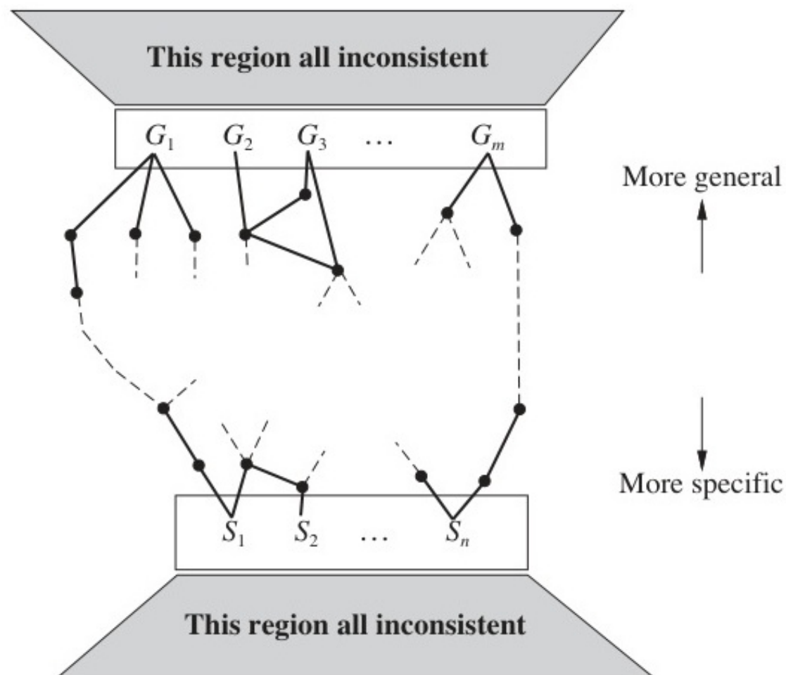
Figure 20.2: Không gian phiên bản chứa tất cả các giả thuyết nhất quán với các ví dụ, nằm giữa hai tập giới hạn G và S .
