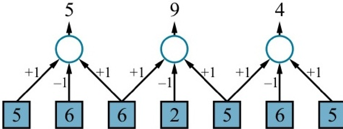
Figure 22.2: Hoạt động của Tích chập (Convolution) trượt bộ lọc qua ảnh để trích xuất đặc trưng.
