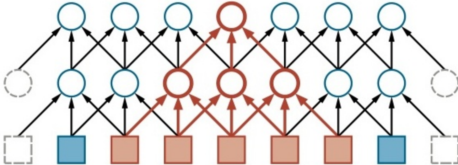
Figure 22.3: Hai tầng đầu tiên của một mạng Nơ-ron Tích chập (CNN) kết nối cục bộ các điểm dữ liệu.
