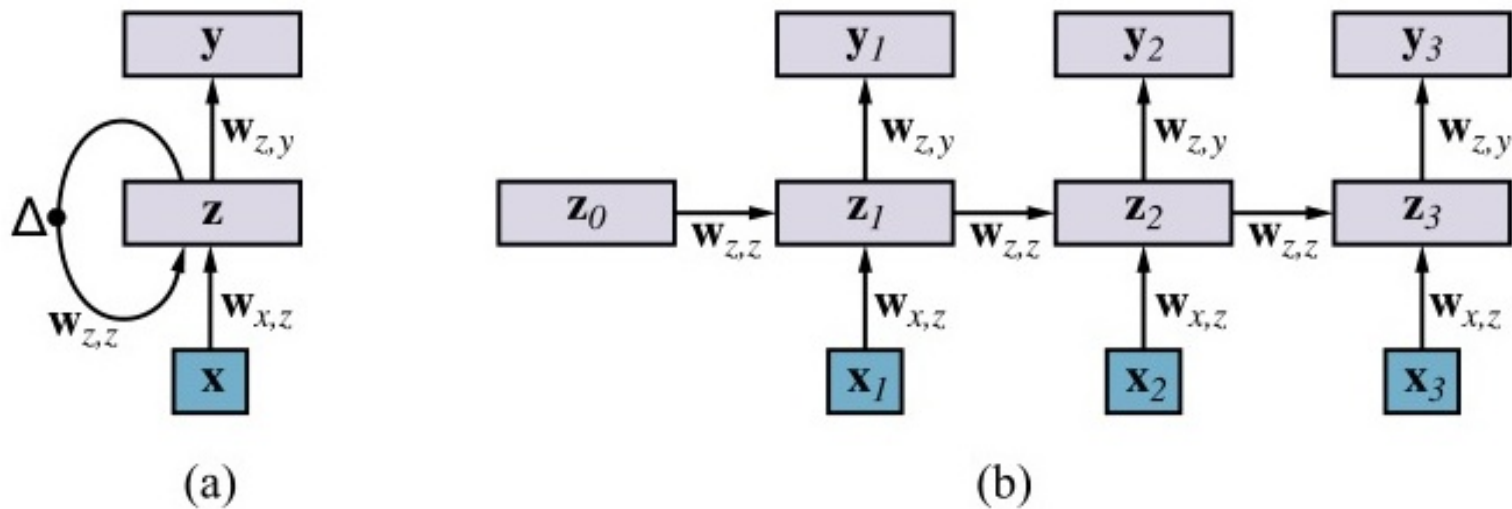
Figure 22.6: Sơ đồ của một Mạng Nơ-ron Hồi quy (RNN) có vòng lặp thời gian truyền trạng thái ẩn.
