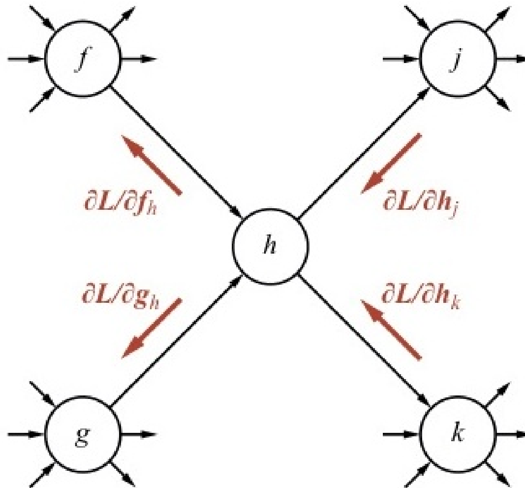
Figure 22.4: Minh họa quá trình Lan truyền ngược (Backpropagation) thông tin gradient trên đồ thị tính toán.
