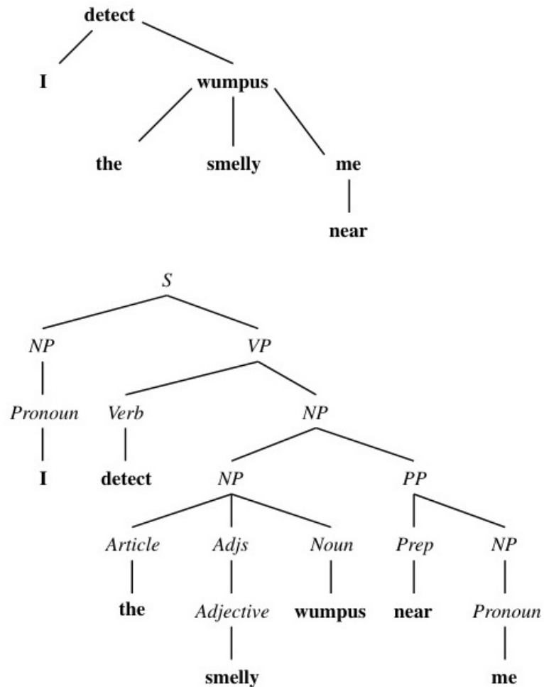
Figure 24.7: So sánh giữa Cây phân tích phụ thuộc (trên) và Cây phân tích cấu trúc cụm từ truyền thống (dưới).
