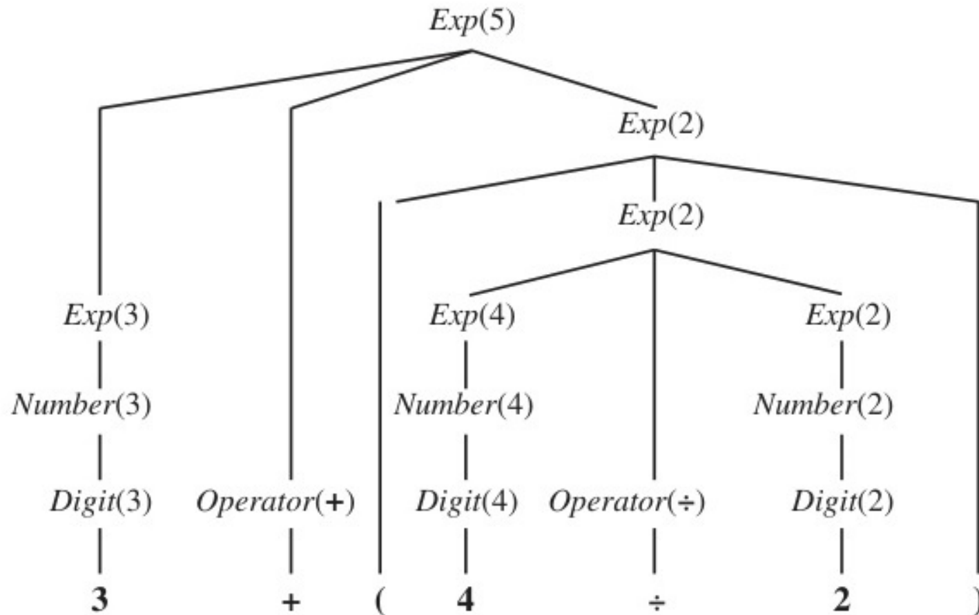
Figure 24.11: Cây phân tích cú pháp kèm diễn giải ngữ nghĩa cho chuỗi 3 + (4 / 2) .
