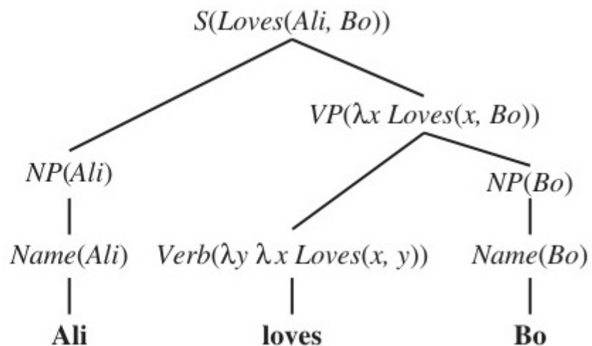
Figure 24.12: Một ngữ pháp đơn giản có khả năng dẫn xuất ra cả Cây phân tích cú pháp lẫn Ý nghĩa logic (Semantics) của một câu.
