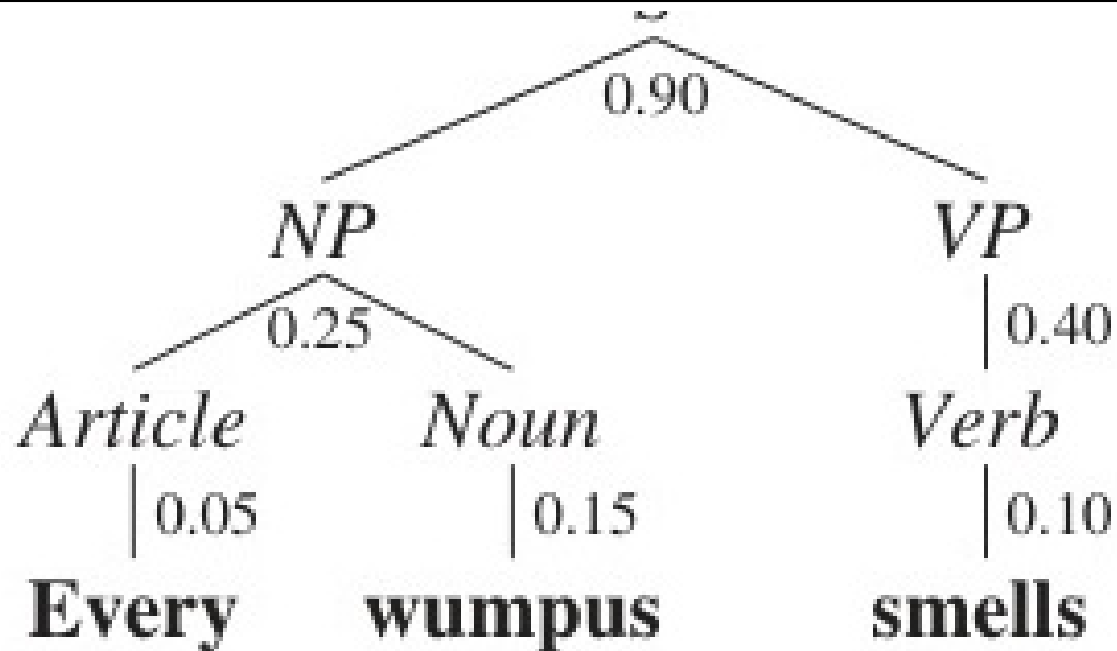
Figure 24.6: Ví dụ về một Cây phân tích cú pháp (Parse Tree) hoàn chỉnh cho một câu tiếng Anh.
