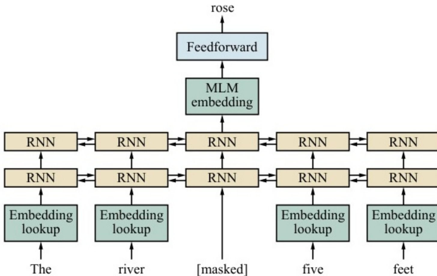
Figure 25.12: Đào tạo mô hình BERT bằng cách che các từ đầu vào và yêu cầu mô hình dự đoán chính xác từ bị che.
