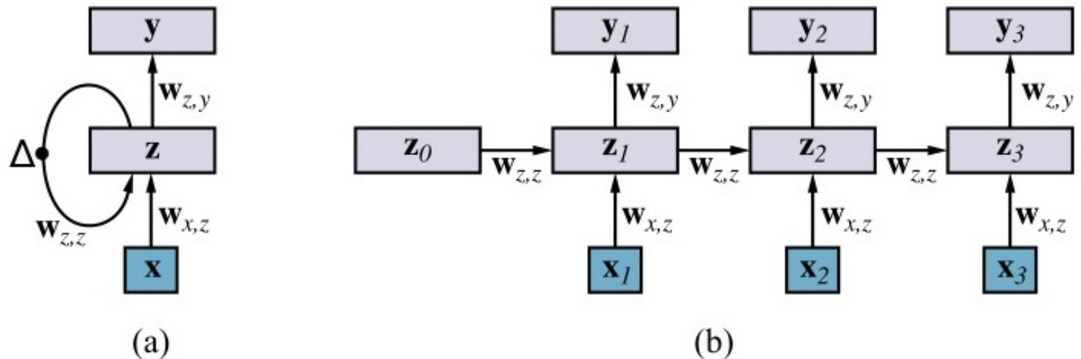
Figure 25.4: Sơ đồ RNN với vòng lặp (trái) và sau khi trải ra theo thời gian (phải) để dự đoán hoặc phân loại.
