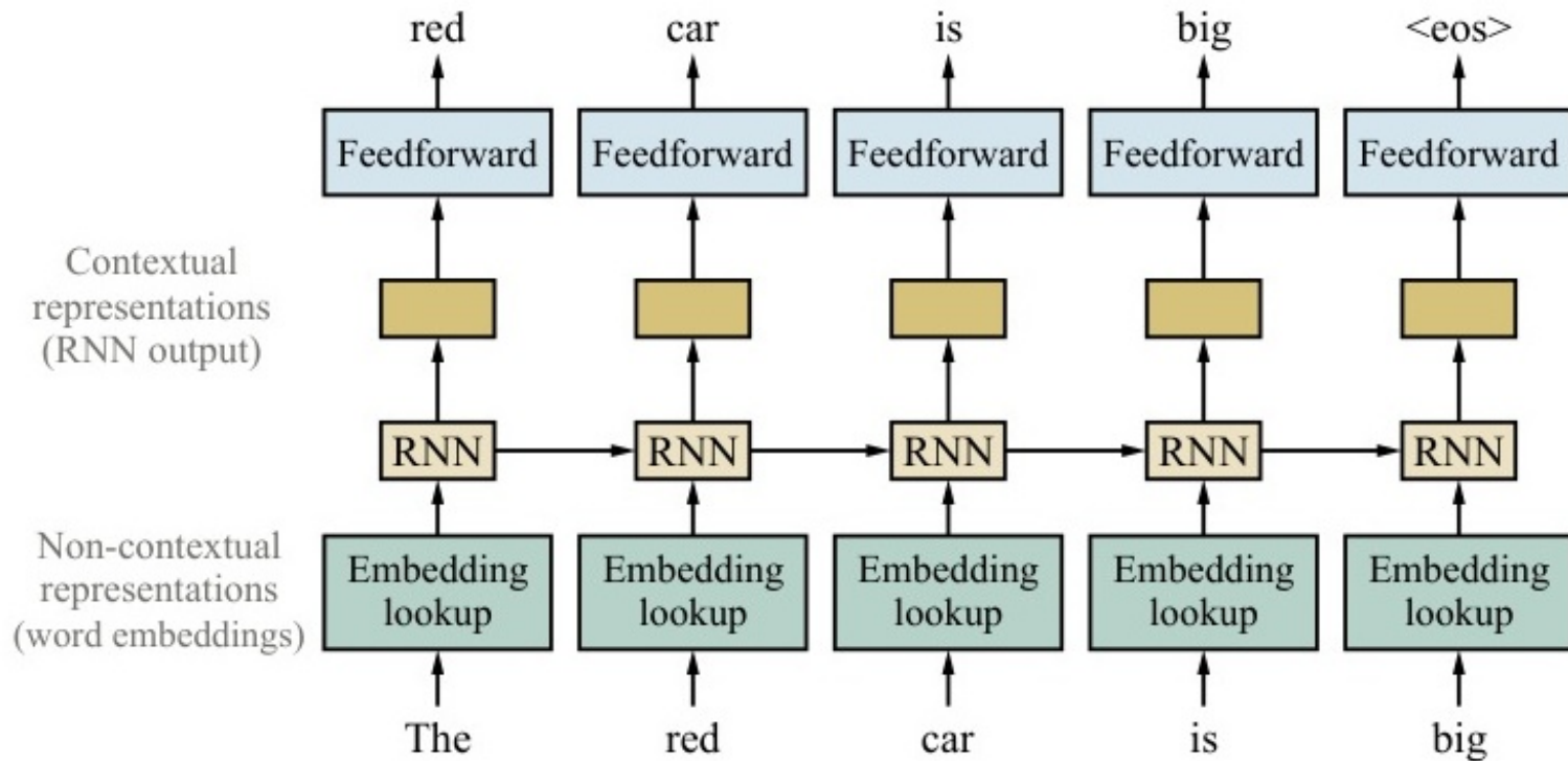
Figure 25.11: Mạng nơ-ron tạo ra nhúng từ có ngữ cảnh, giúp phân biệt ý nghĩa của từ dựa vào các từ xung quanh.
