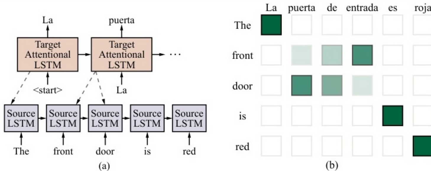
Figure 25.7: Cơ chế chú ý giúp mô hình tập trung linh hoạt vào các phần khác nhau của câu nguồn qua hàm xác suất Softmax.
