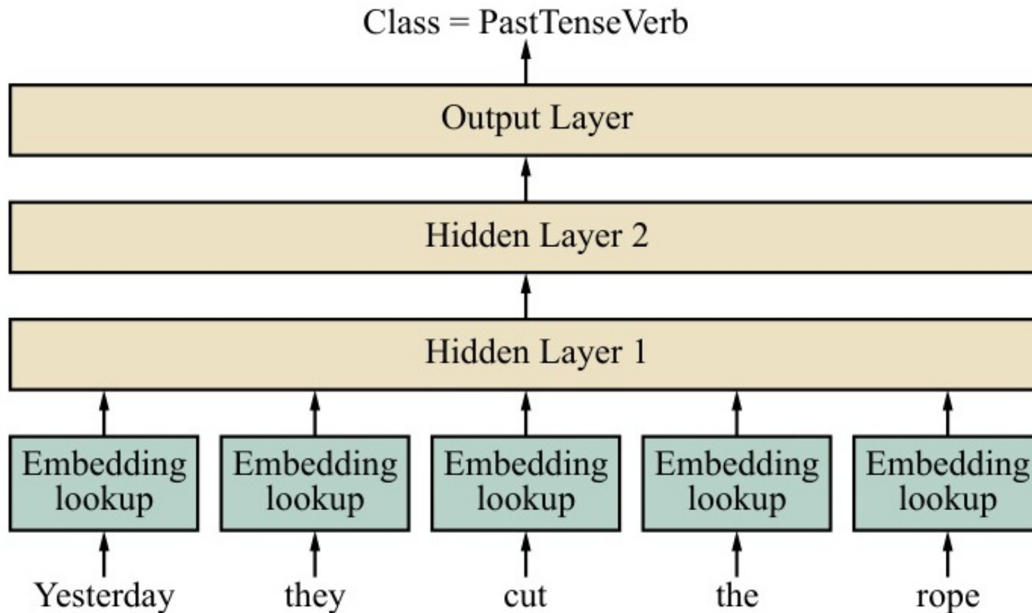
Figure 25.3: Cấu trúc mạng nơ-ron truyền thẳng xuất ra nhãn từ loại từ một cửa sổ văn bản, kết hợp ma trận nhúng từ.
