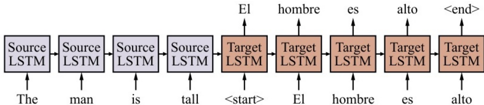
Figure 25.6: Cấu trúc Seq2Seq cơ bản với LSTM dịch từ "The man is tall" sang ngôn ngữ đích.
