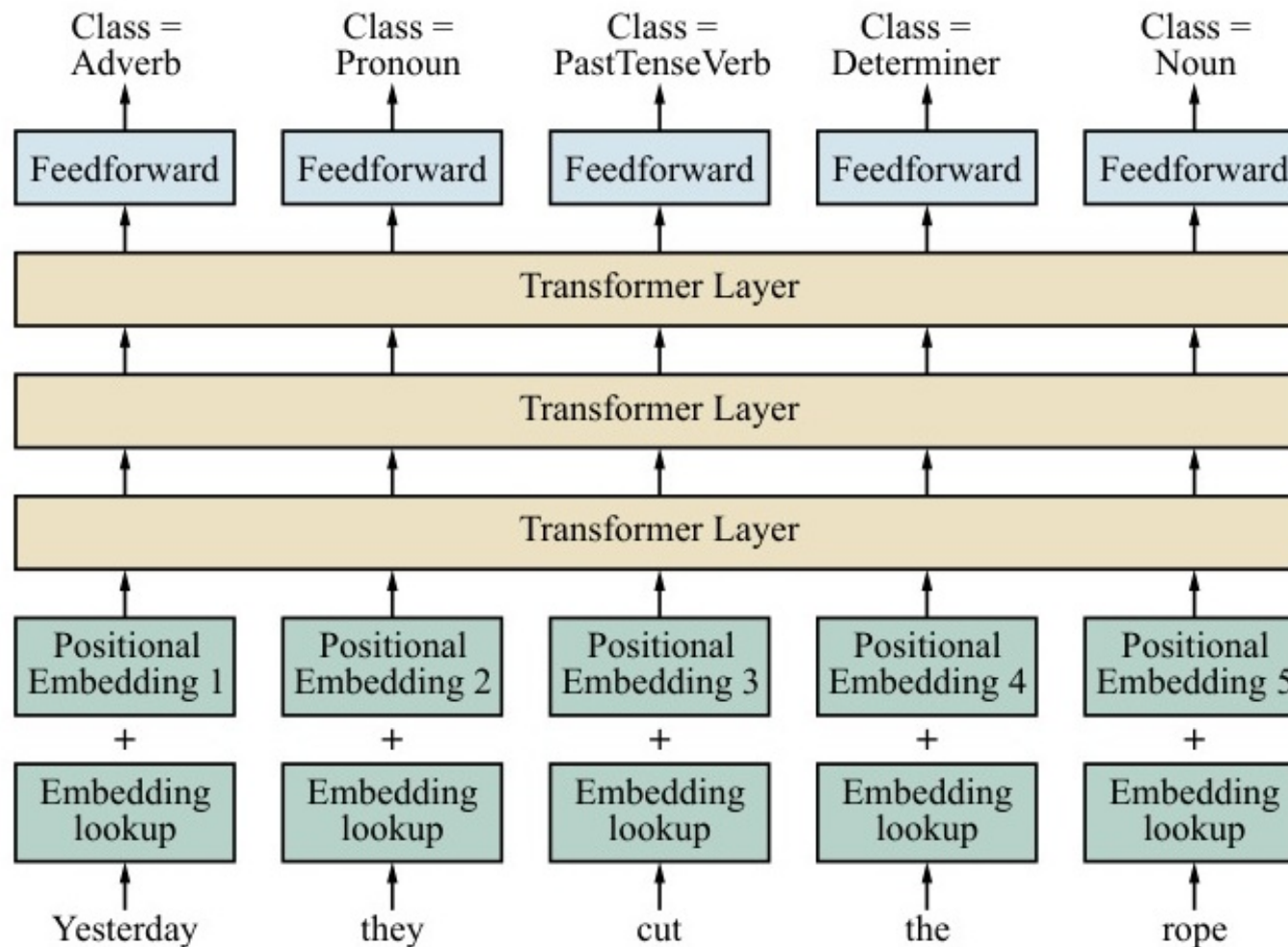
Figure 25.10: Sử dụng kiến trúc Transformer để thực hiện Gán nhãn Từ loại (POS Tagging).
