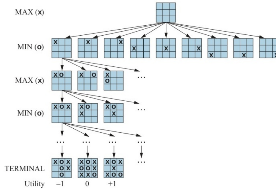
Figure 1: Mô phỏng 2 nước đi đầu tiên trong cây trò chơi Cờ caro (Tic-Tac-Toe).
