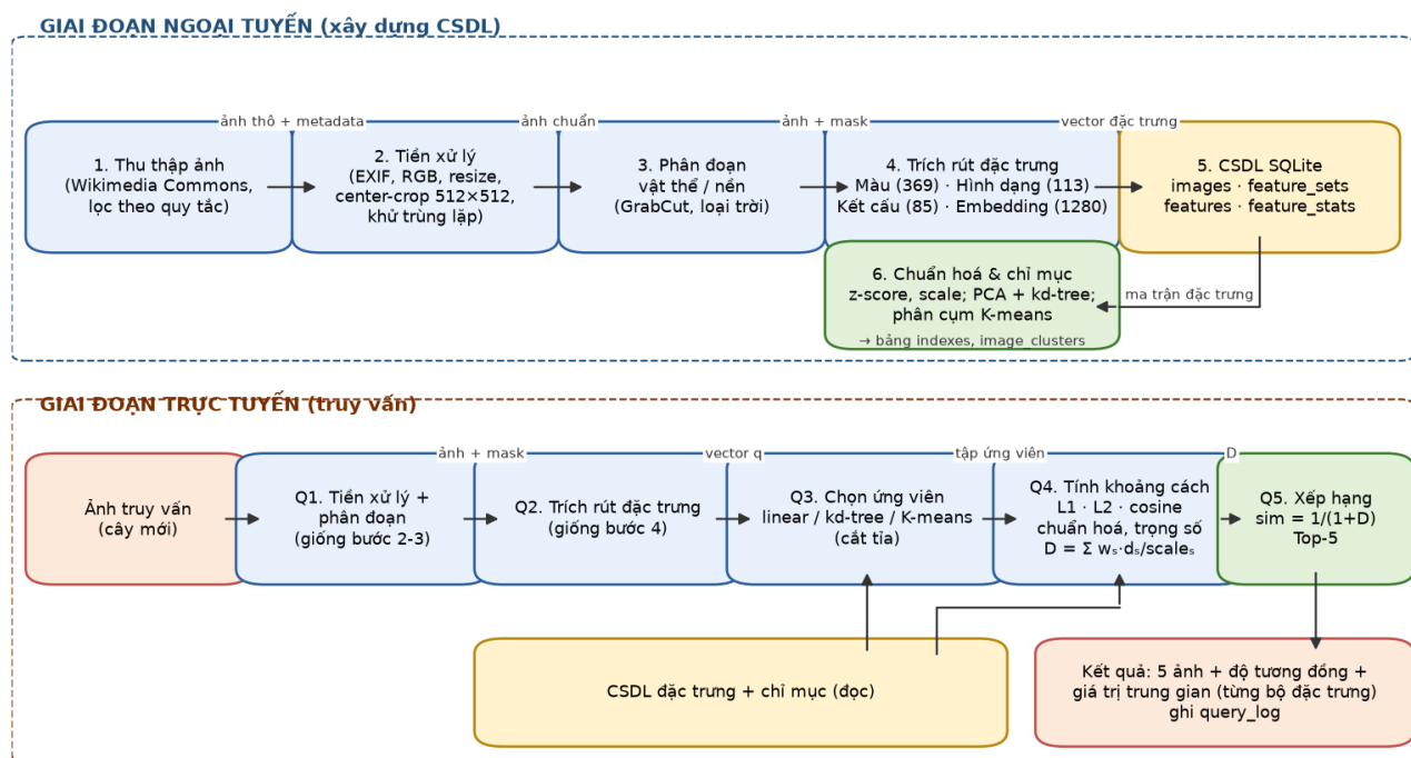
Hình 6. Sơ đồ khối hệ thống: giai đoạn ngoại tuyến (trên) và trực tuyến (dưới)
