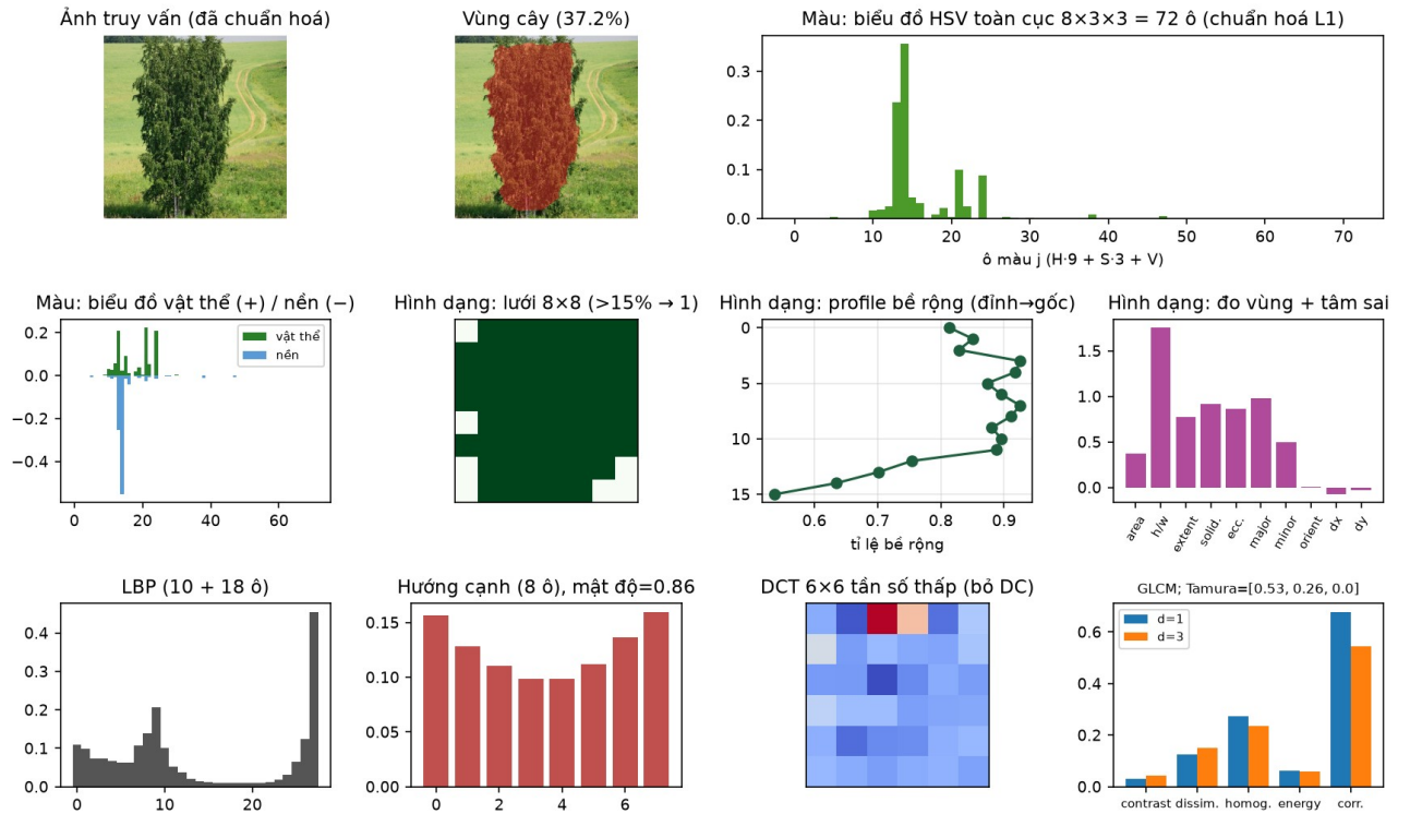
Hình 7. Biểu diễn trực quan các đặc trưng của ảnh truy vấn query_01.jpg
