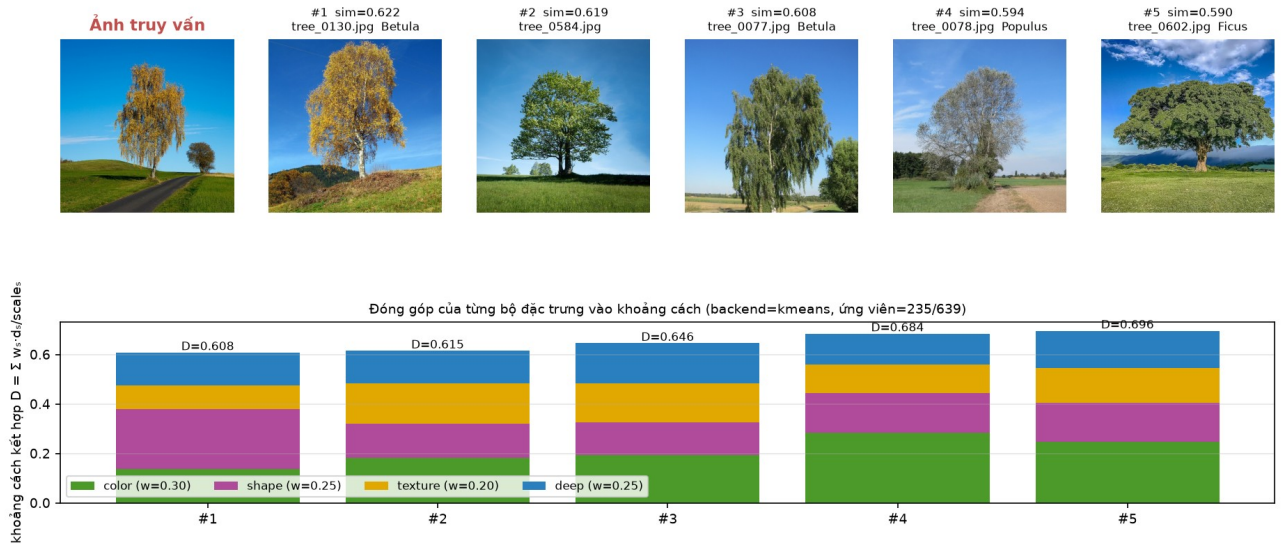
Hình 12. Kết quả top-5 cho ảnh query_04.jpg (backend kmeans)
