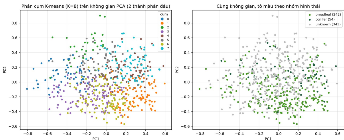
Hình 5. Phân bố ảnh trong không gian PCA: theo cụm K-means (trái) và theo nhóm hình thái (phải)
