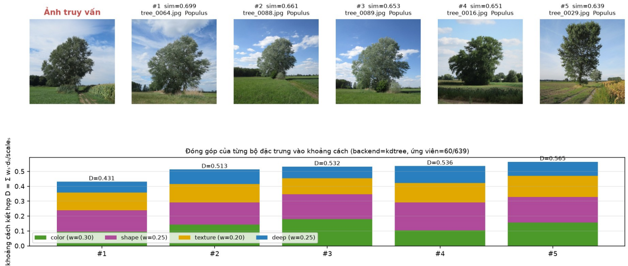
Hình 11. Kết quả top-5 cho ảnh query_03.jpg (backend kdtree)
