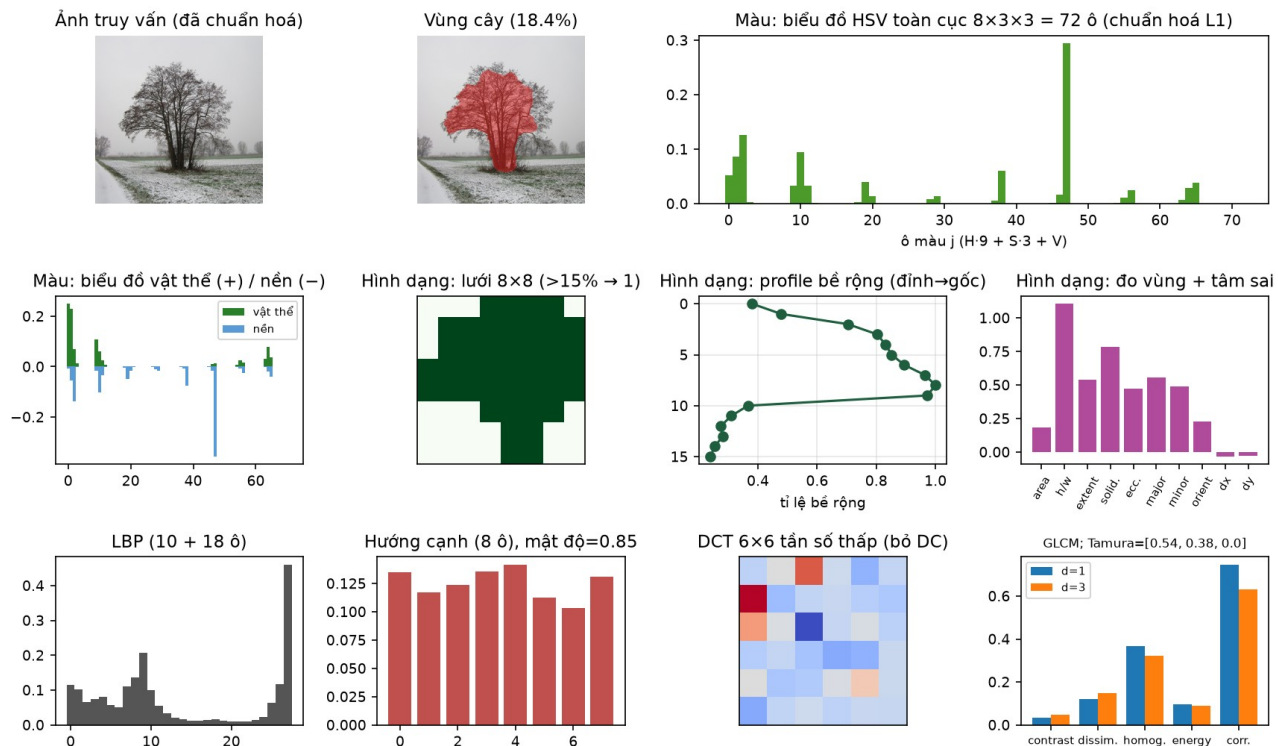
Hình 9. Biểu diễn trực quan các đặc trưng của ảnh truy vấn query_02.jpg
