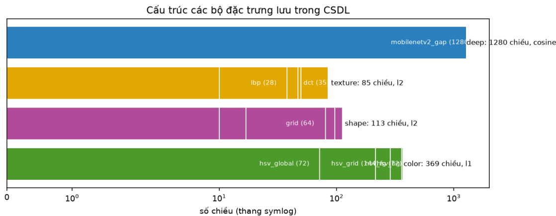
Hình 3. Cấu trúc các khối trong từng bộ đặc trưng lưu trong CSDL
