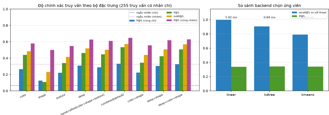
Hình 13. Độ chính xác theo bộ đặc trưng (trái) và so sánh backend (phải)
