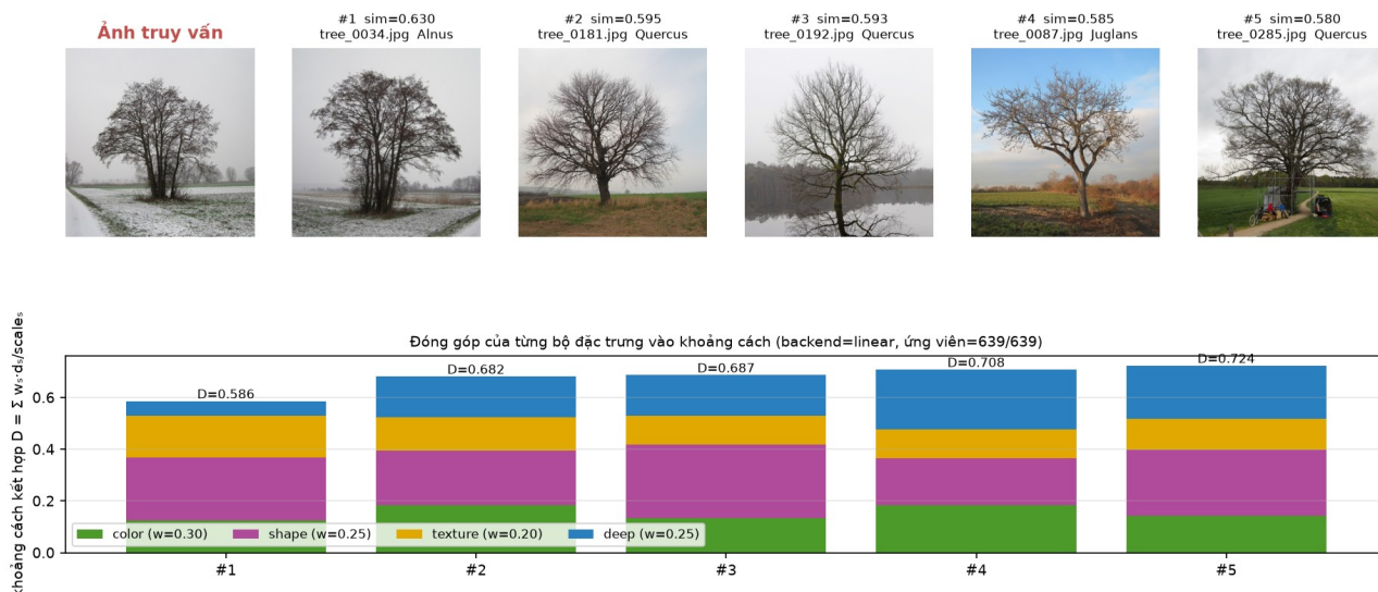
Hình 10. Kết quả top-5 cho ảnh query_02.jpg và đóng góp của từng bộ đặc trưng vào khoảng cách kết hợp
