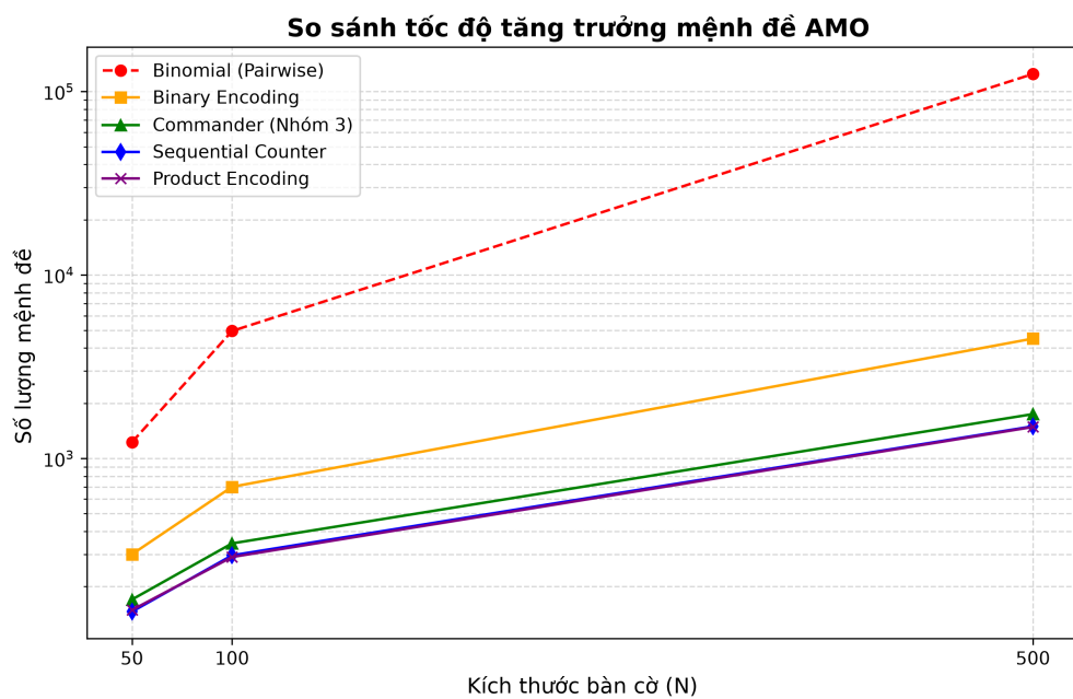
Hình 1: Biểu đồ so sánh tốc độ tăng trưởng số lượng mệnh đề của các phương pháp AMO (thang đo Logarit).
