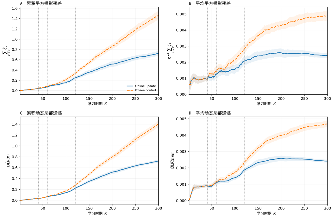
图 5-4 缓变环境中的连续在线跟踪
