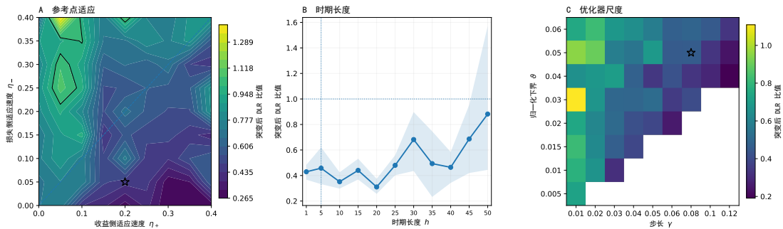
图 5-5 参考点机制消融及在线跟踪优势的稳健性
