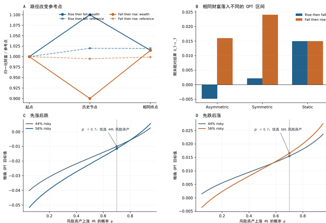
图 5-2 财富路径、参考点与投资组合选择
