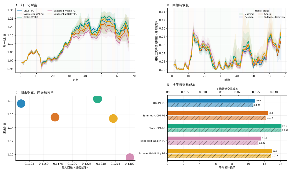
图 5-6 A 股时间顺序回放中的财富、回撤与交易成本
