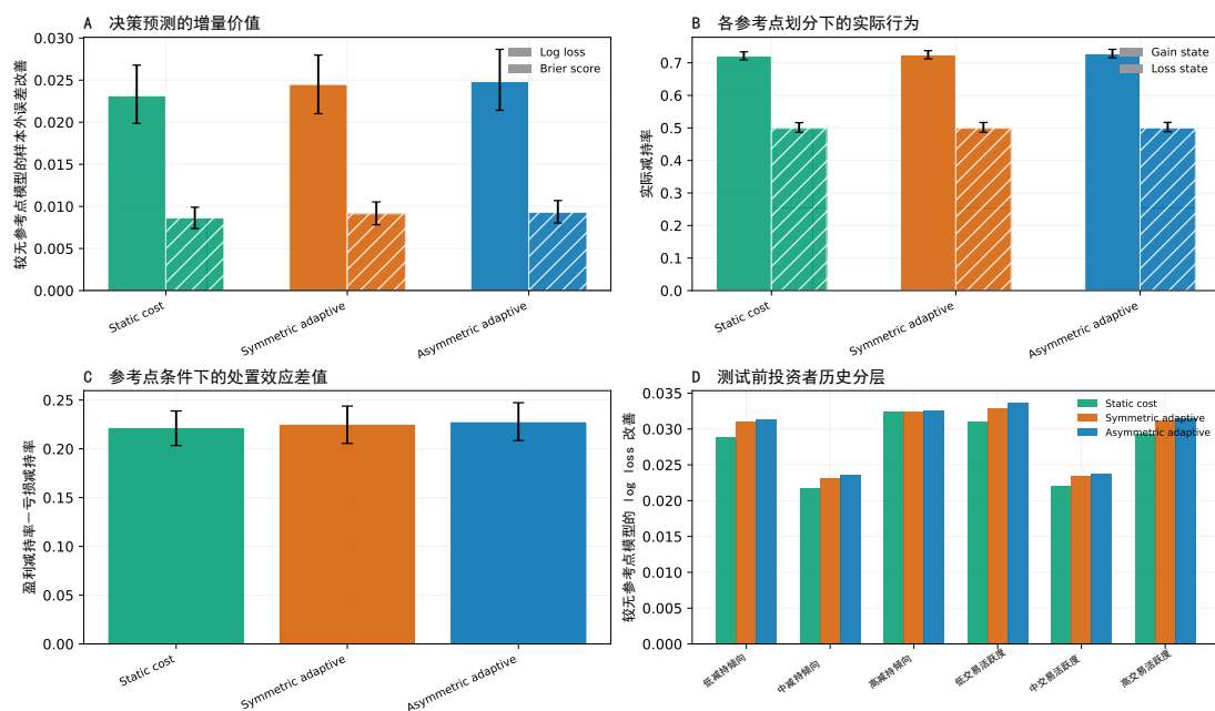
图 5-7 参考点与投资者减持行为的样本外比较
