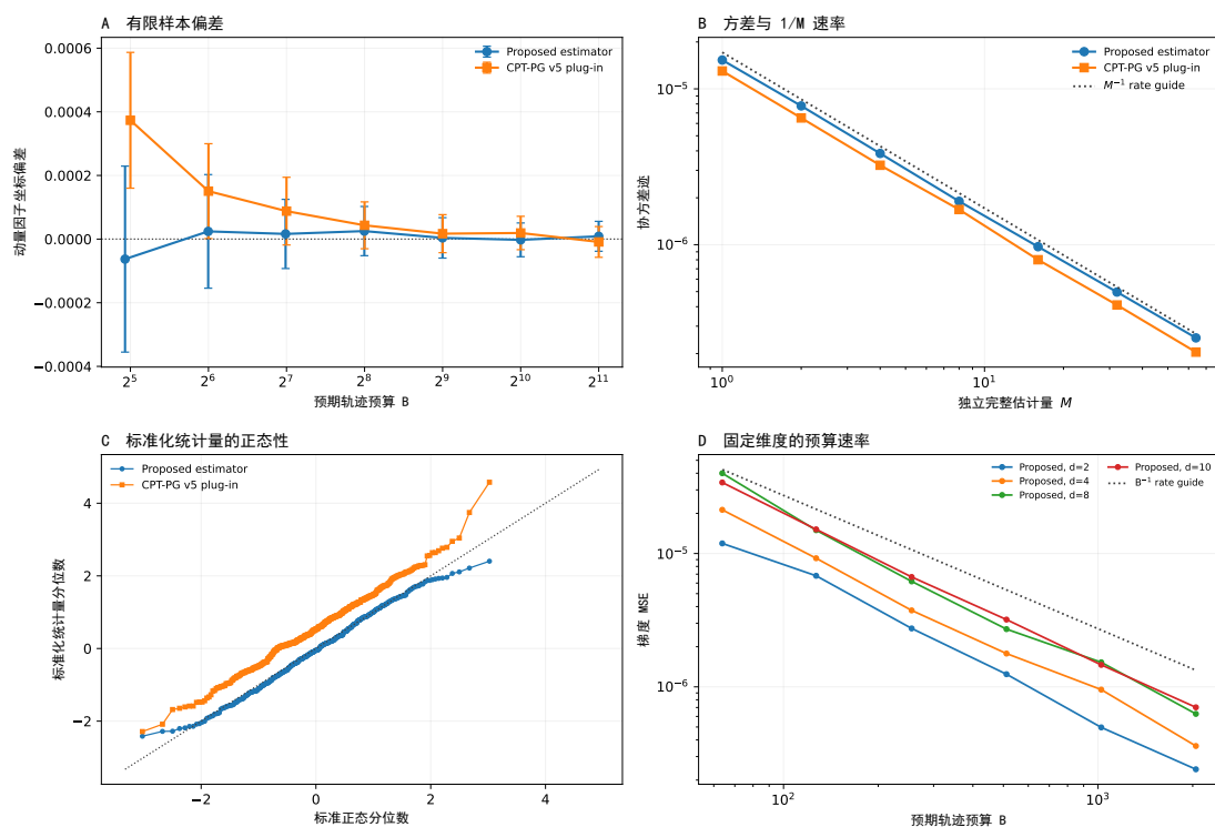
图 5-3 半合成环境中的有限样本梯度估计
