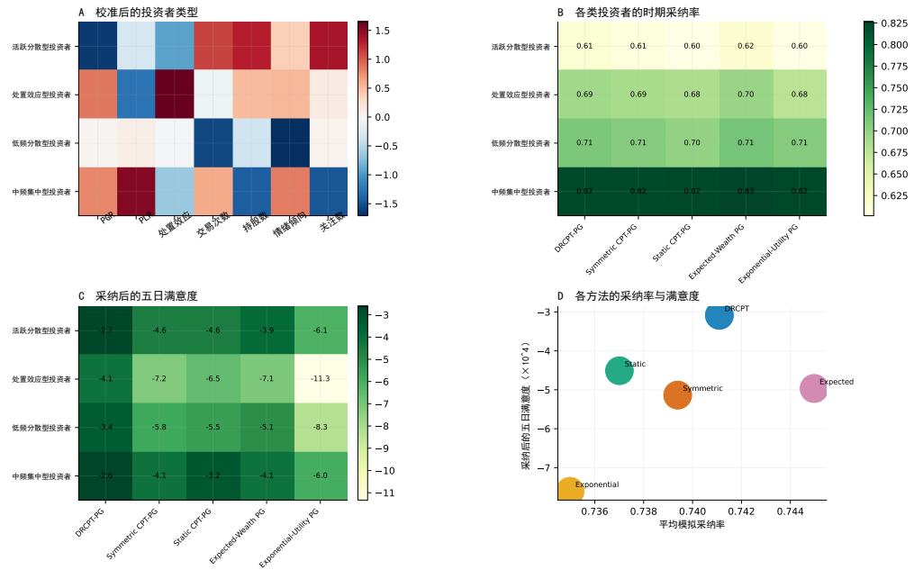
图 5-8 异质投资者的持续模拟交互
