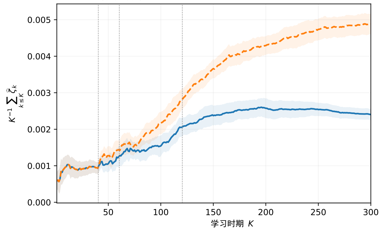
D 平均动态局部遗憾
