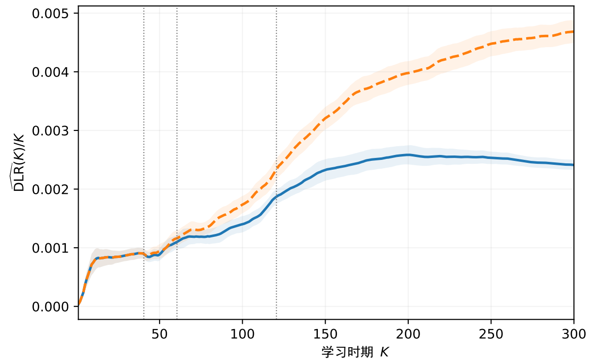
D 平均动态局部遗憾
