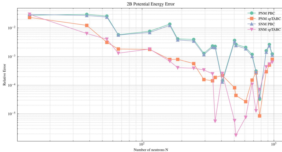
Figure 3.1: In figura è rappresentato l’errore di una simulazione del ground state di un sistema di molti fermioni che interagiscono tramite termini a due e a tre corpi. Le diverse simulazioni sono state eseguite per sistemi di materia puramente neutronica (PNM) e di materia simmetrica (SNM), ciascuna approssimando il ground state di Hartree-Fock usando condizioni periodiche al contorno (PBC) o quasi-periodiche (Twist Angle Boundary Conditions). Il twist angle viene usato per minimizzare l’errore nel passaggio al limite termodinamico: funge, in pratica, da regolarizzatore.
