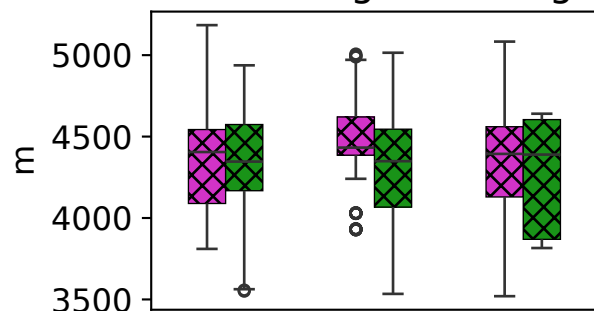
Min. melting level height
