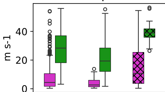
Max. updraft
