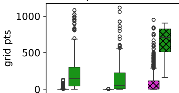
Updraft area
