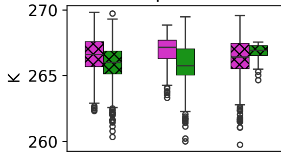
Min. temp. at 500 hPa
