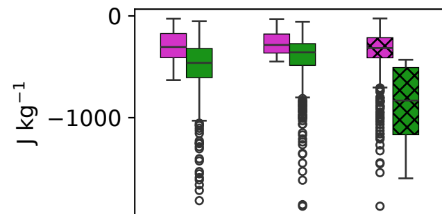
Min. CIN
