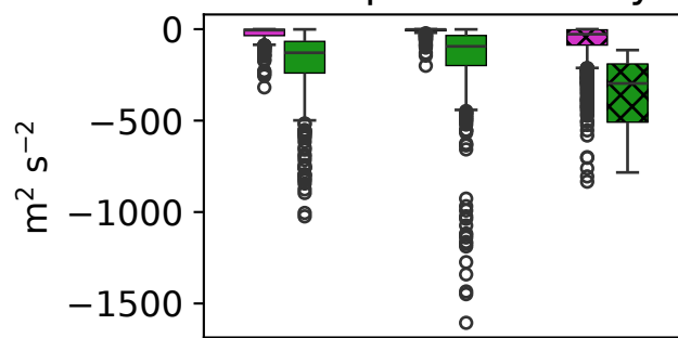
Min. updraft helicity
