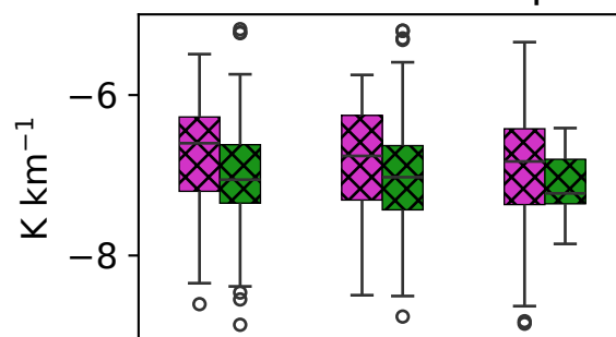
Min. 700 to 500 hPa lapse rate
