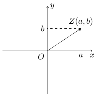
图 1-2: 复数 z
