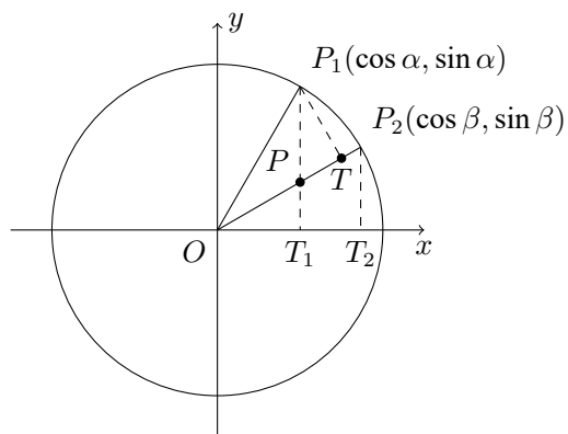
图 2-1: \begin{cases} \sin(\alpha - \beta) = \sin \alpha \cos \beta - \sin \beta \cos \alpha \\ \cos(\alpha - \beta) = \cos \alpha \cos \beta + \sin \alpha \sin \beta \end{cases} 的几何证明
