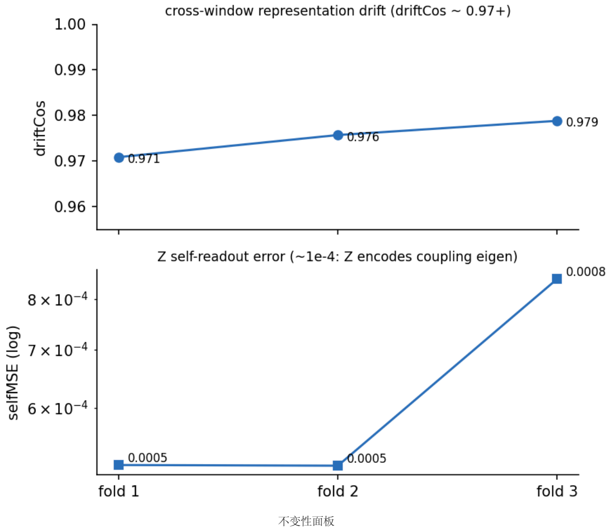
图 5 — 不变性面板：跨窗口表示稳定性（漂移余弦 \approx 0.97 ）与精华自治 MSE。全部主结果使用的无头配置下，selfMSE 跨折为 0.0005–0.0008；融合预测头下膨胀至 0.0008–0.0496（附录 D）。
