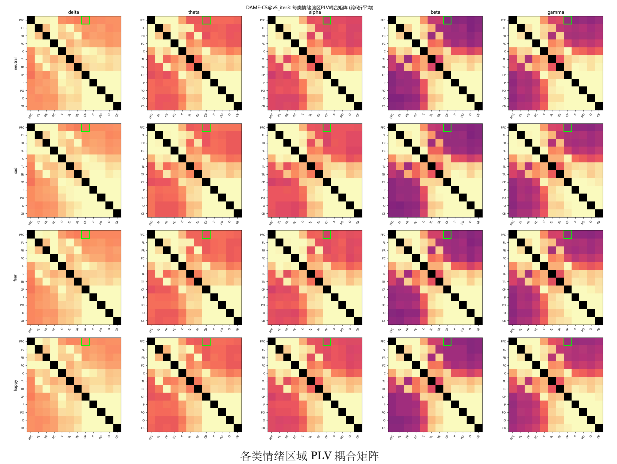
图 2a — 各类情绪区域 PLV 耦合矩阵（第3轮，折平均）：4 情绪类 × 5 频段。全局结构跨类不变（第 VI-E 节 P3），配对级差异集中在 DMN 轴上。
