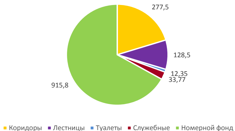
Соотношение площадей типового этажа, м 2
