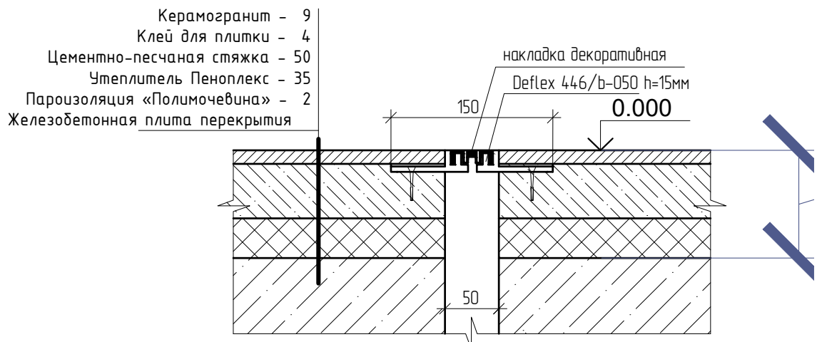
Узел 1. Устройства деформационного шва. М 1:5 (принципиальная схема)
