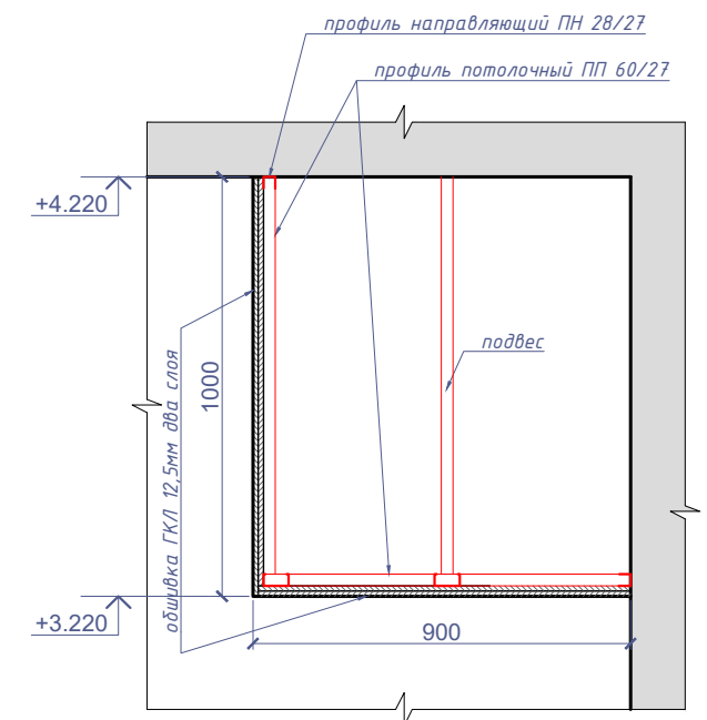
Сечение 3-3 (М1:20)
