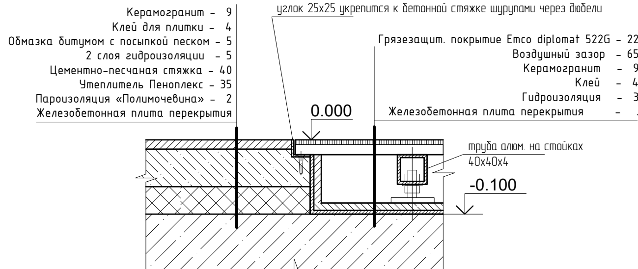
Узел 2. Углубления для грязезащитного покрытия. М 1:5
