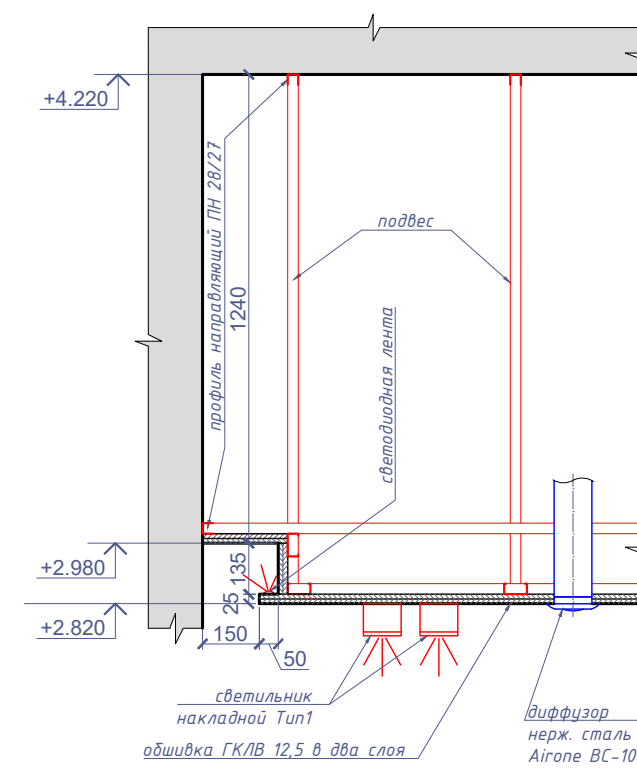
Сечение 3-3 (М1:20)
