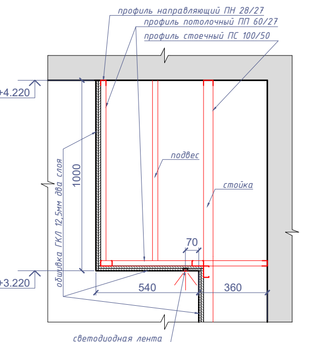
Сечение 4-4 (М1:20)
