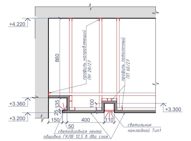
Сечение 2-2 (М1:20)
