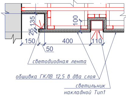
Узел 1 (М1:20)
