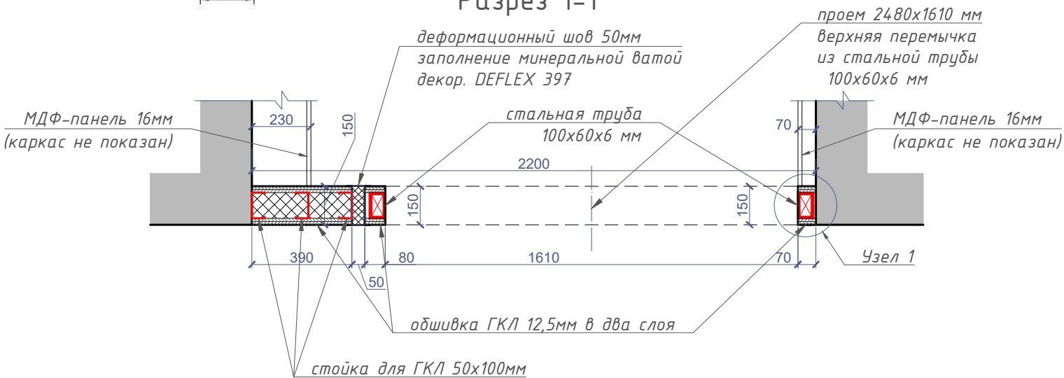
Разрез 1-1
