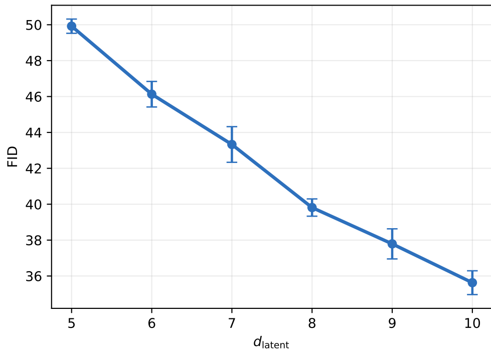
FID
