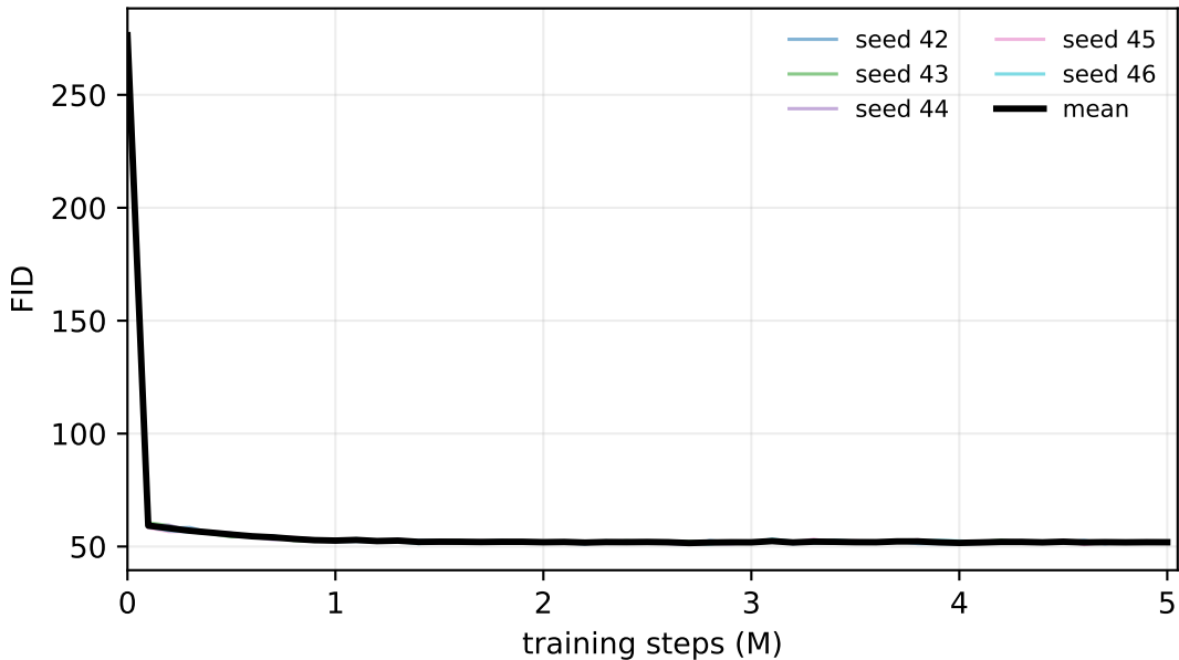
CelebA d=40
