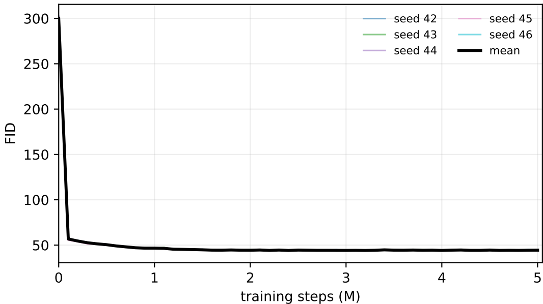
CelebA d=60
