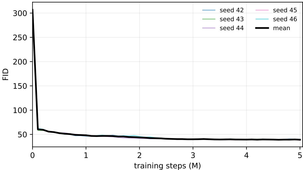
CelebA d=90
