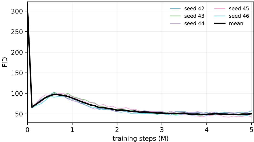
CelebA d=200
