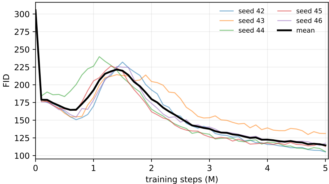
CIFAR-10 d=120
