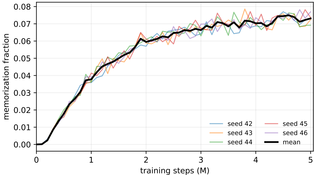
CIFAR-10 d=40
