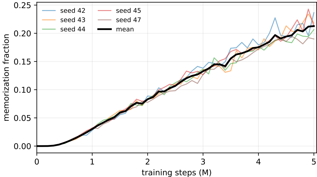
CIFAR-10 d=220
