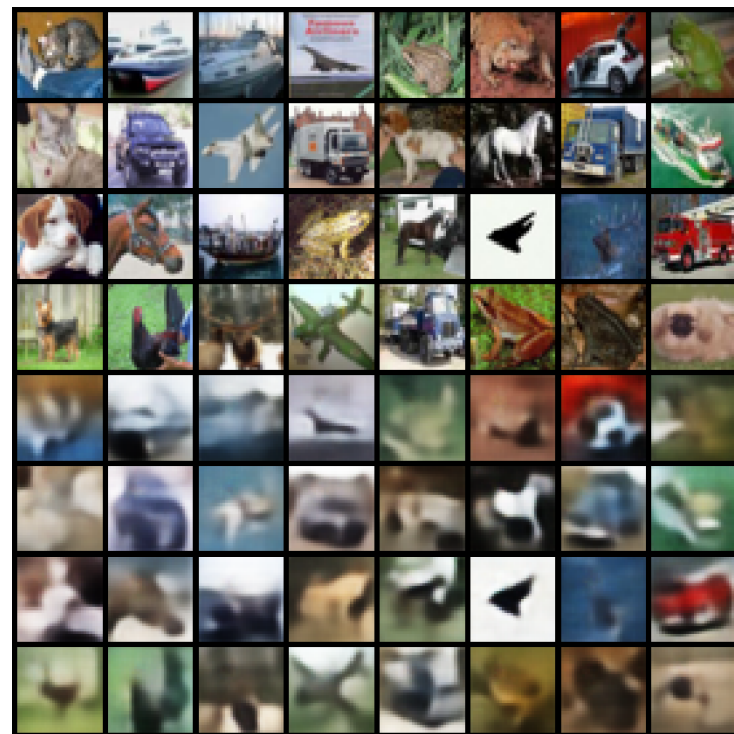
d_{latent} = 160
