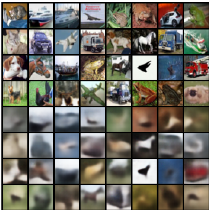
d_{latent} = 100
