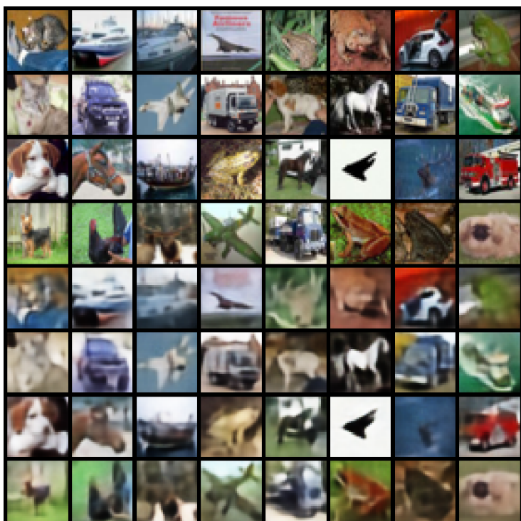
d_{latent} = 220
