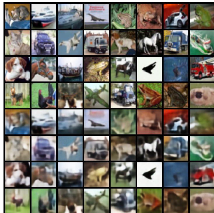
d_{latent} = 260
