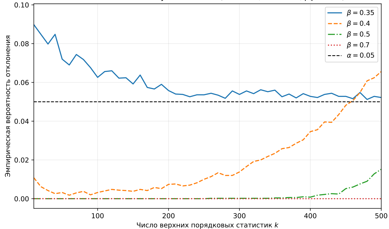
Степенные хвосты: нулевой класс ( n = 2500 , B = 5000 , \beta_0 = 0.35 )
