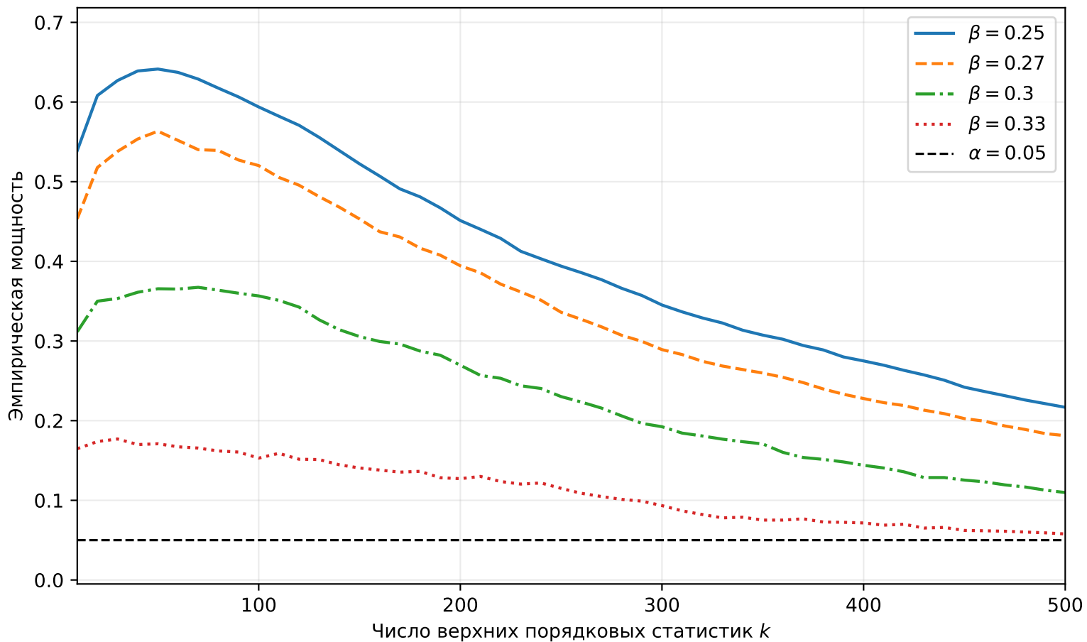
Степенные хвосты: альтернативный класс ( n = 2500 , B = 5000 , \beta_0 = 0.35 )
