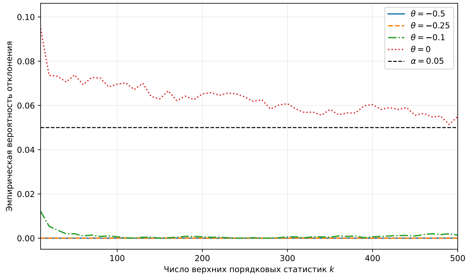
Логарифмически возмущенные хвосты: нулевой класс ( n = 2500 , B = 5000 )
