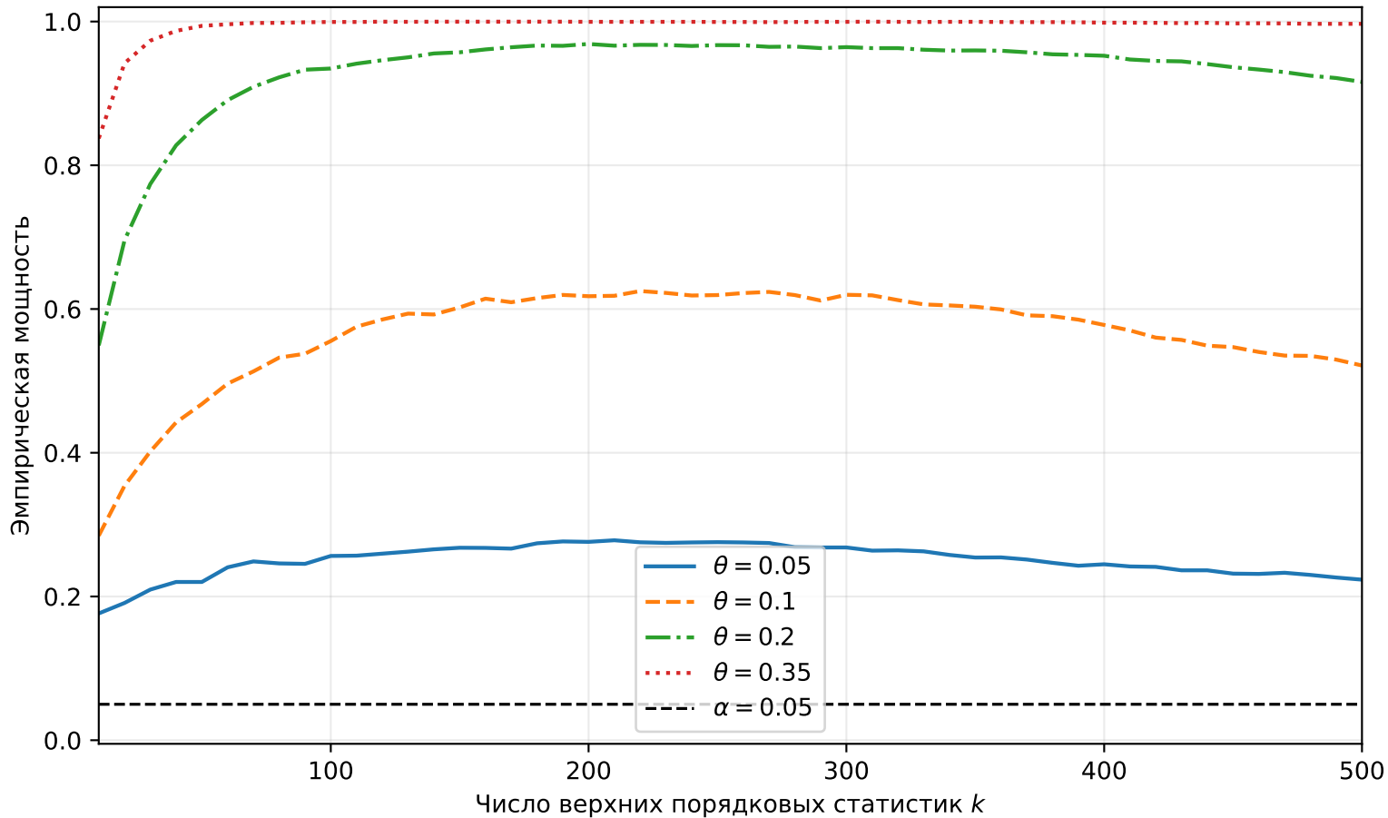
Логарифмически возмущенные хвосты: альтернативный класс ( n = 2500 , B = 5000 )
