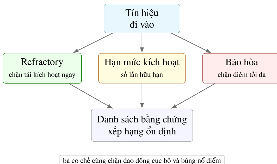
Hình 3.13: Ba cơ chế bảo vệ chu trình
