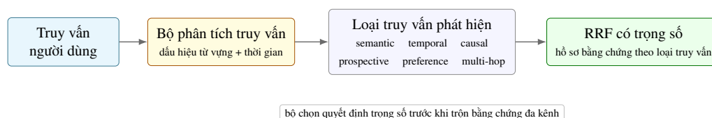
Hình 3.14: Adaptive Query Routing
