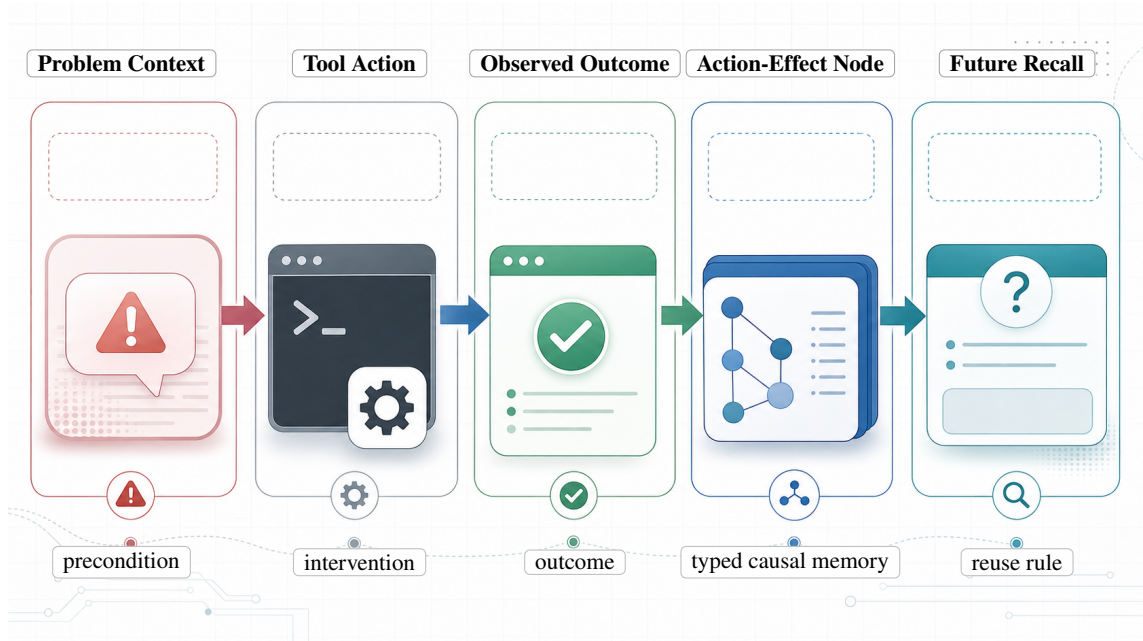
Figure 4.5: Action-effect phù hợp với trace AI agent thật, nơi hệ thống cần nhớ quan hệ giữa điều kiện lỗi, hành động tool và kết quả quan sát được.
