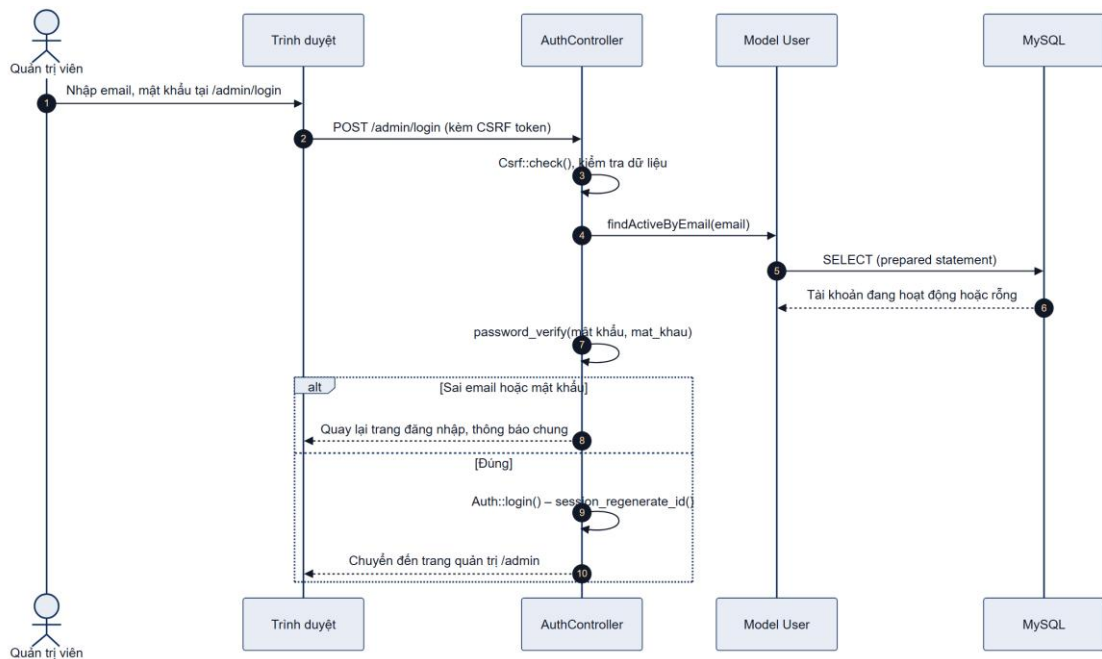
Hình 3.5. Sơ đồ tuần tự chức năng đăng nhập quản trị
