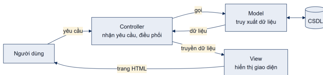
Hình 2.2. Mô hình Model – View – Controller
