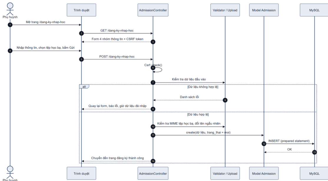
Hình 3.4. Sơ đồ tuần tự chức năng đăng ký nhập học
