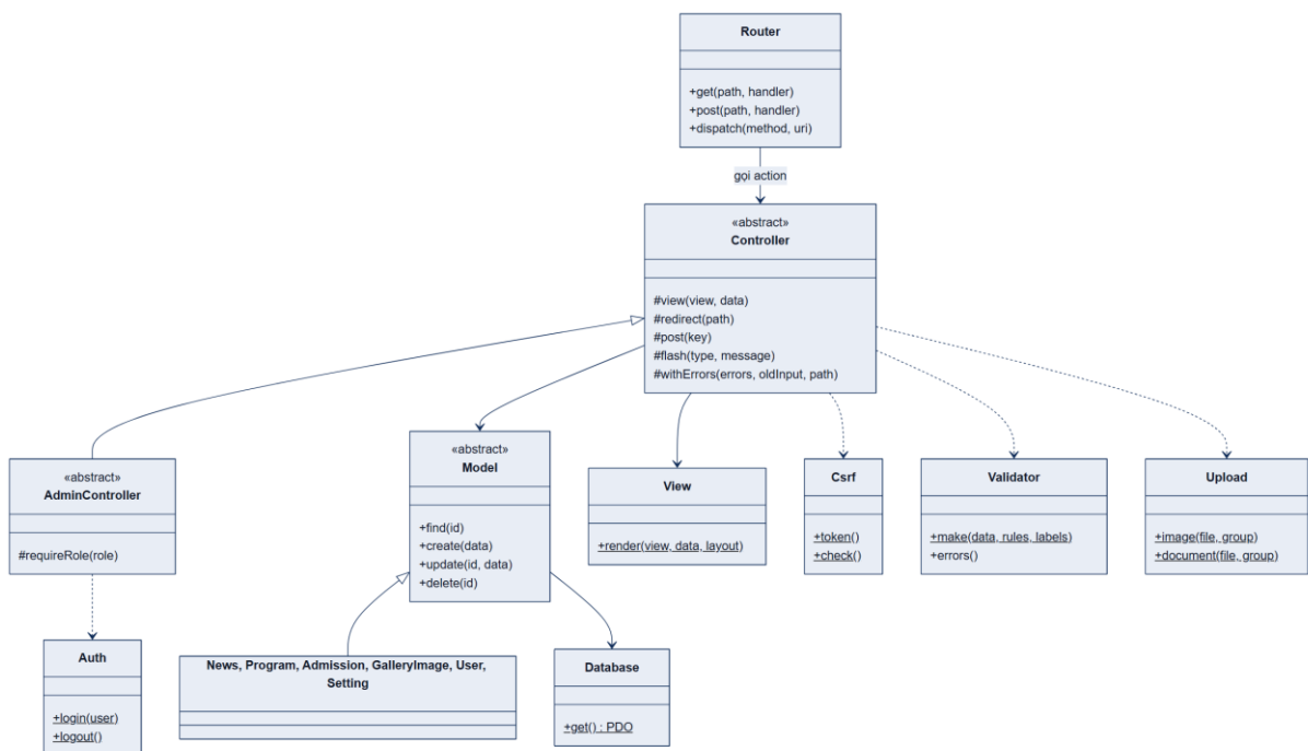
Hình 3.2. Sơ đồ lớp các thành phần lỗi
