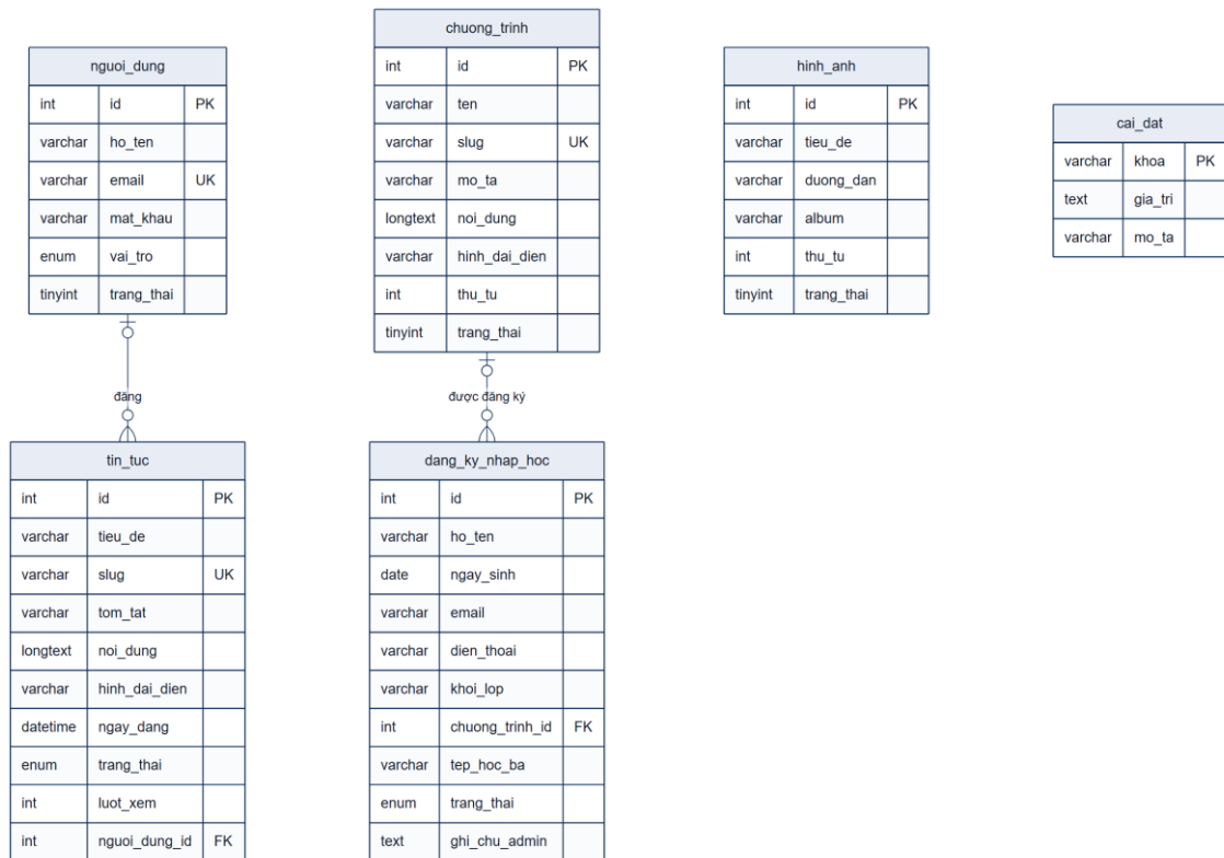
Hình 3.8. Sơ đồ ERD của cơ sở dữ liệu
