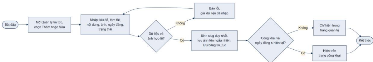
Hình 3.7. Sơ đồ hoạt động quản lý tin tức
