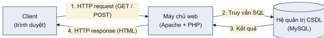
Hình 2.1. Mô hình client – server
