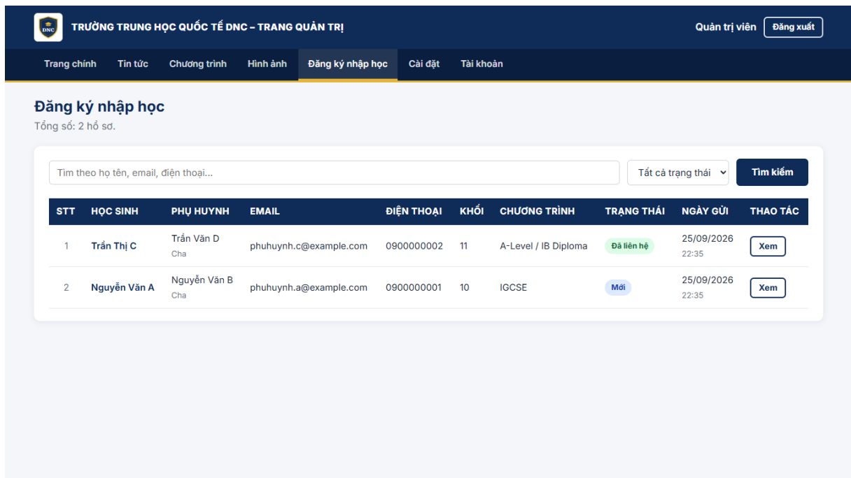
Hình 4.21. Danh sách hồ sơ đăng ký
