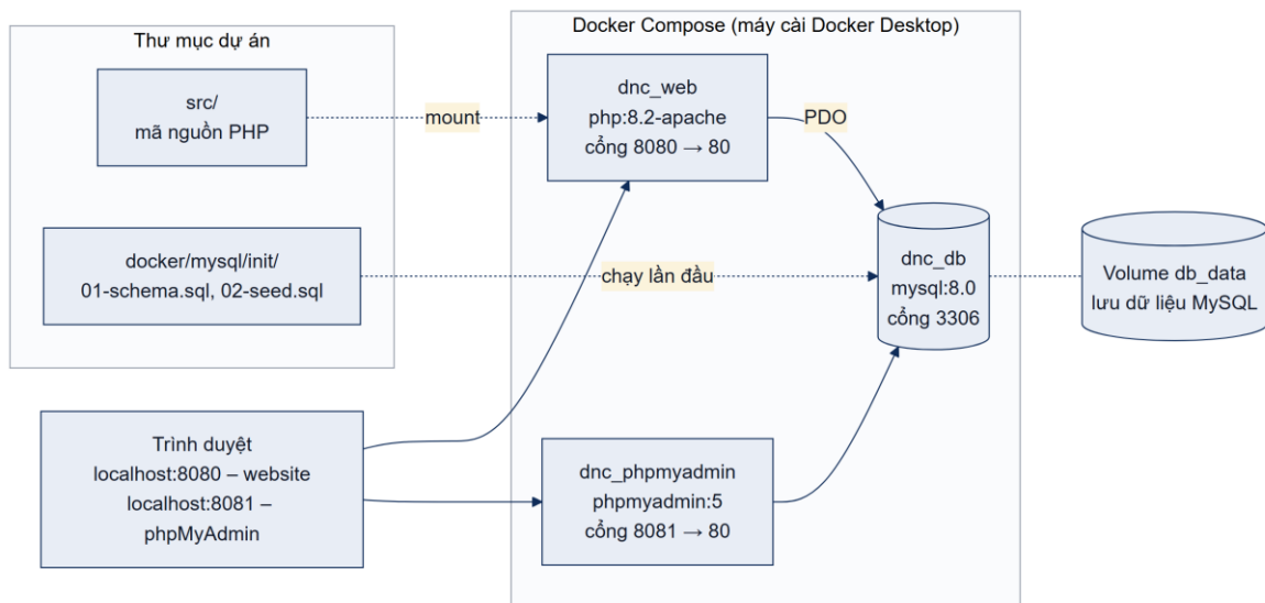
Hình 3.9. Sơ đồ triển khai bằng Docker Compose
