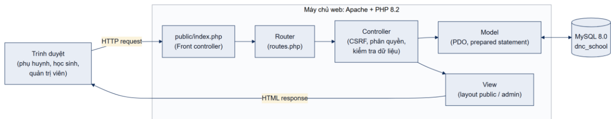
Hình 3.1. Kiến trúc tổng quát của hệ thống
