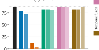
(f) UniVLA
