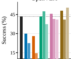
OpenVLA
