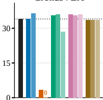
CronusVLA
