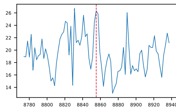
041ad37c \lambda=8855.2 S/N=8, lm*
