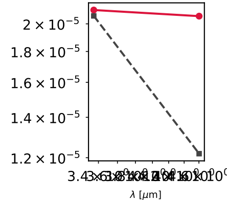
WD 4835613003216896128 Teff=5946K
