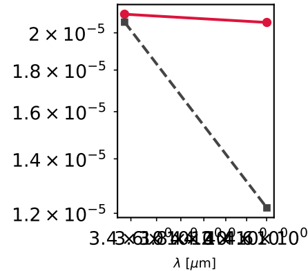
WD 4835613003216896128 Teff=5946K
