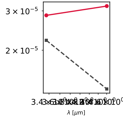
WD 1216861541736356224 Teff=4953K
