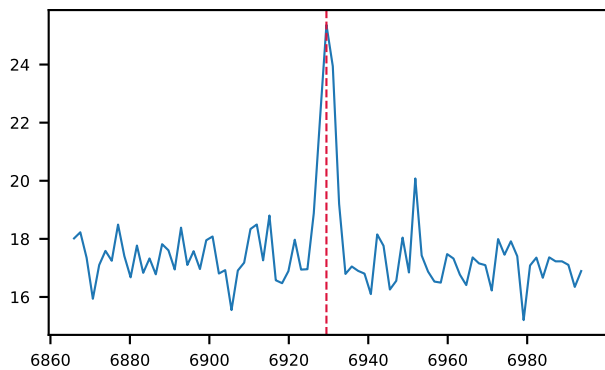
05fc1ec0 \lambda=7490.3 S/N=10, lm*
