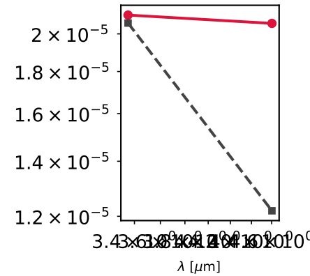
WD 4835613003216896128 Teff=5946K
