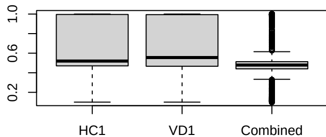
VAF
