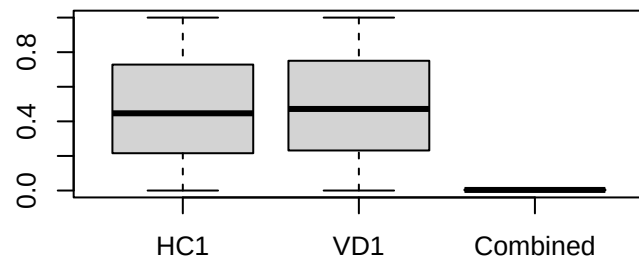
MGRB_AF
