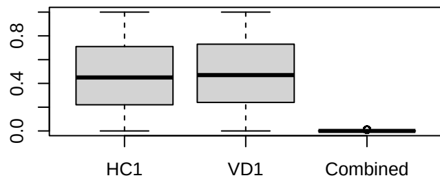
gn_AF
