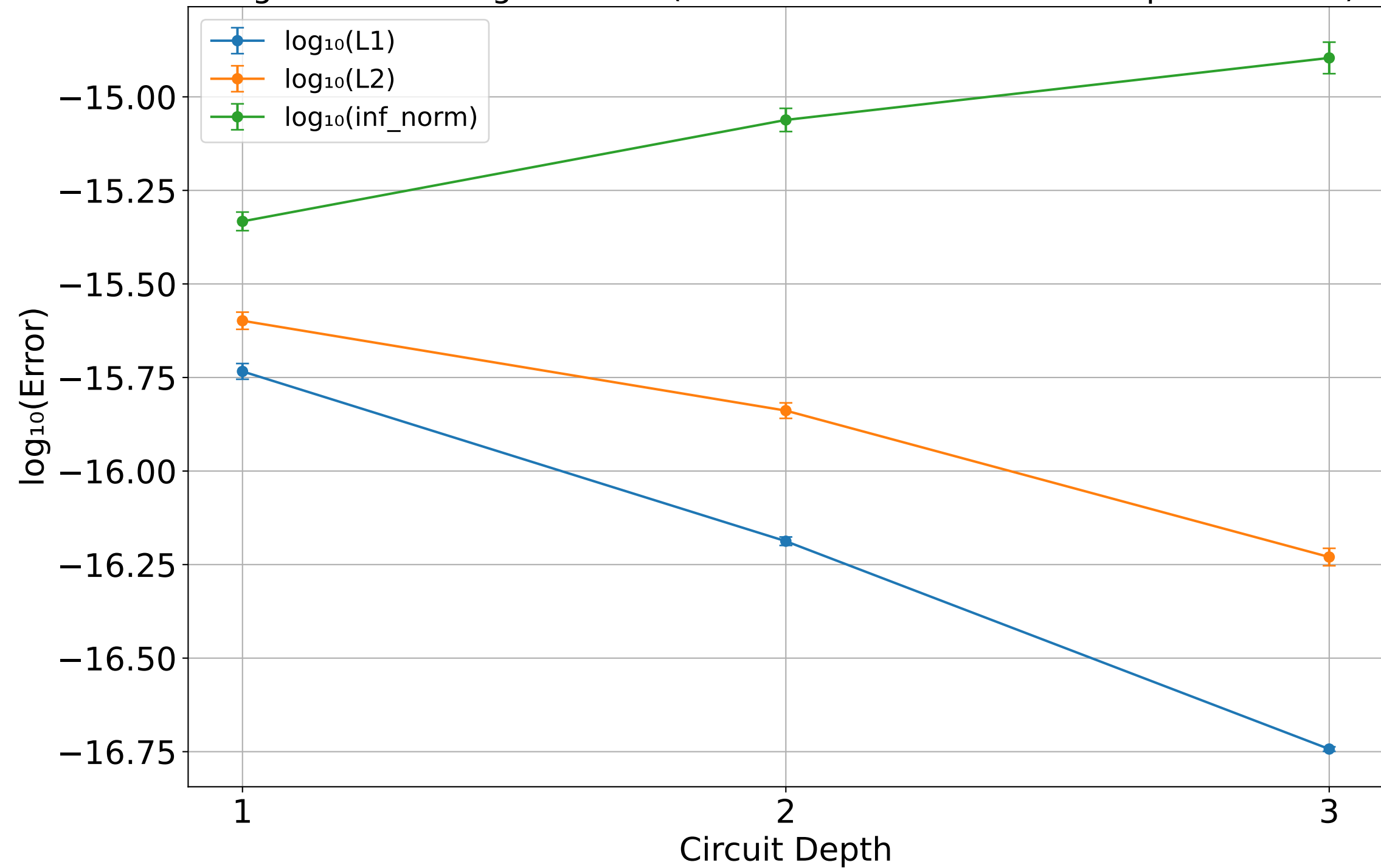
Log-scaled Averaged Errors (over 100 Haar random 300-qubit circuits)
