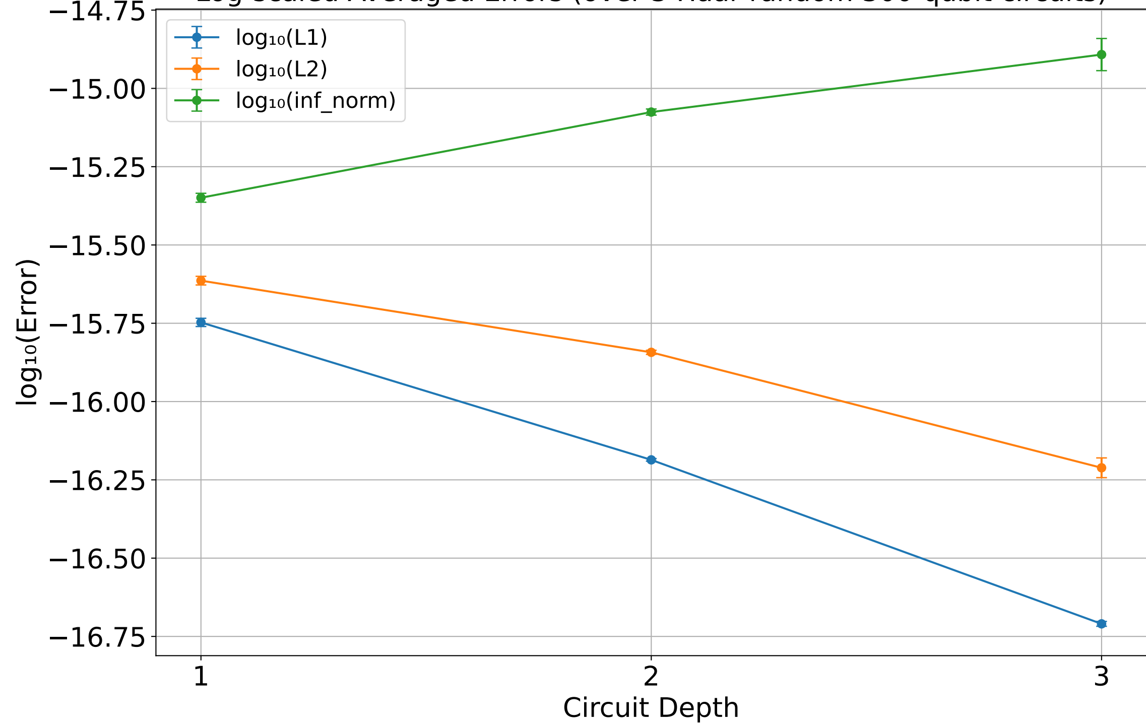
Log-scaled Averaged Errors (over 3 Haar random 300-qubit circuits)
