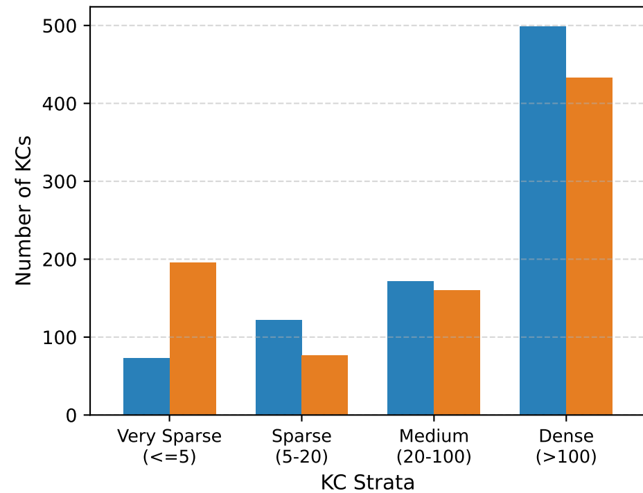
XES3G5M
