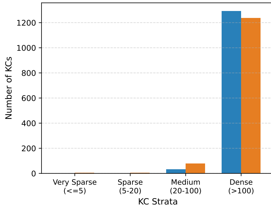
Junyi Academy
