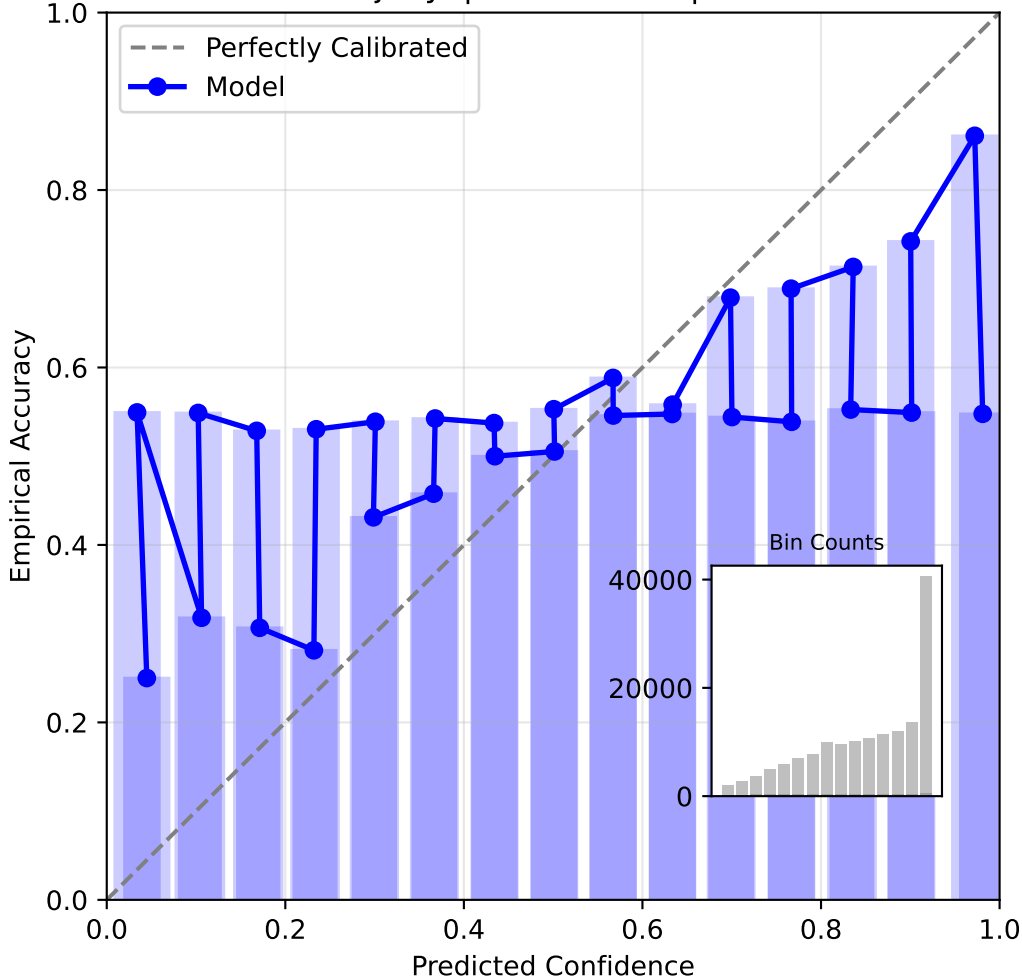
Reliability Diagram: simplekt (medium) Dataset: junyi | ECE: 0.2640 | N: 151597
